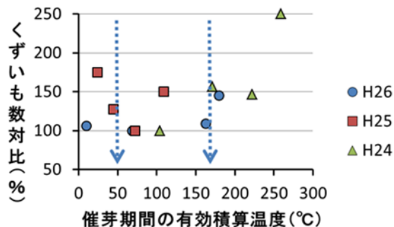
図1 催芽期間の有効積算温度とくずいも数 注) くずいも数対比は各年のくずいも数が最も少ない処理区を100としたときの比で示す。点線はくずいも数から判断した有効積算温度の下限と上限。オホーツク沿海地域における植付時期の有効積算温度は、1週間で約50℃である。
