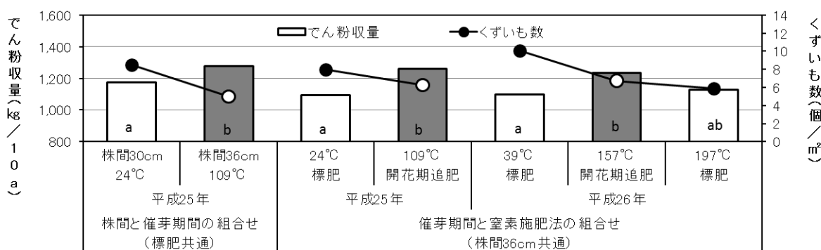
図2 催芽期間、株間、窒素施肥法の最適化がでん粉収量とくずいも数に与える効果(北見農試、普通掘) 注) 同一年次内の異なるアルファベット処理間に有意差あり(5%水準、t検定あるいはTukey法)。 横軸ラベルの温度は催芽期間の有効積算温度。
