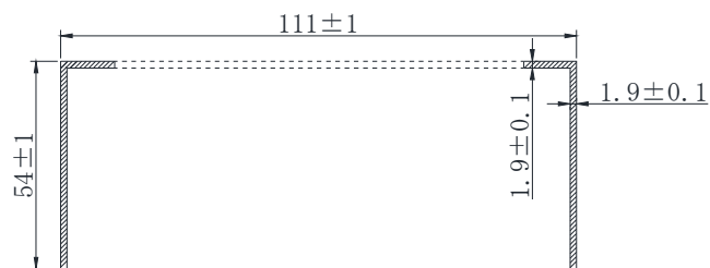
押さえ枠(B-B'断面図)
