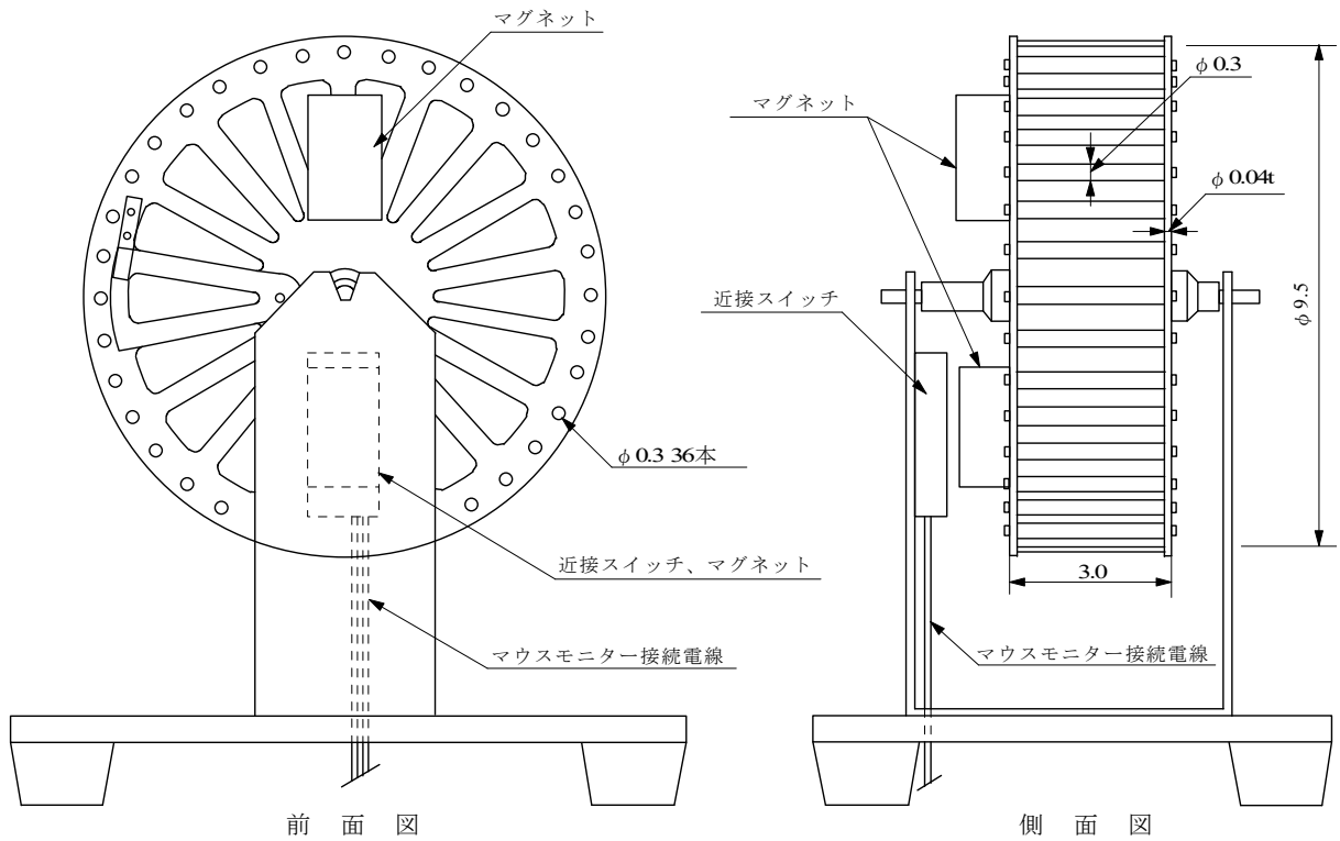
別図9 ガス有害性試験装置の回転かご（寸法単位：cm）（ろ）（ほ）
