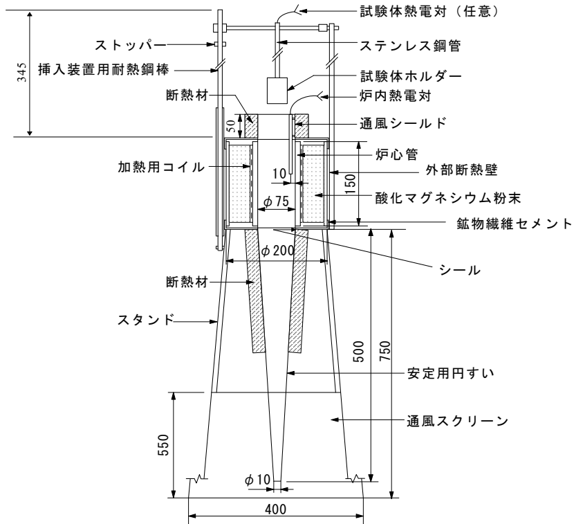
別図1 不燃性試験装置の加熱炉（寸法単位：mm）（ほ）
