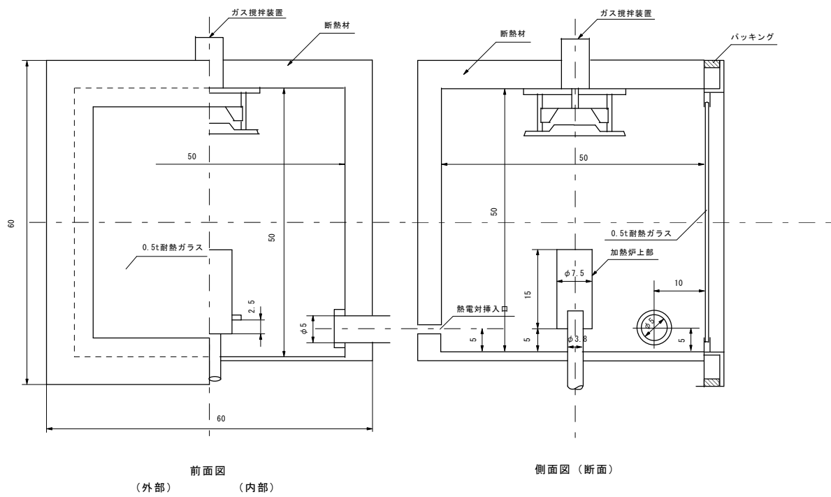
別図7 ガス有害性試験装置の攪拌箱 (寸法単位: cm) (ほ)
