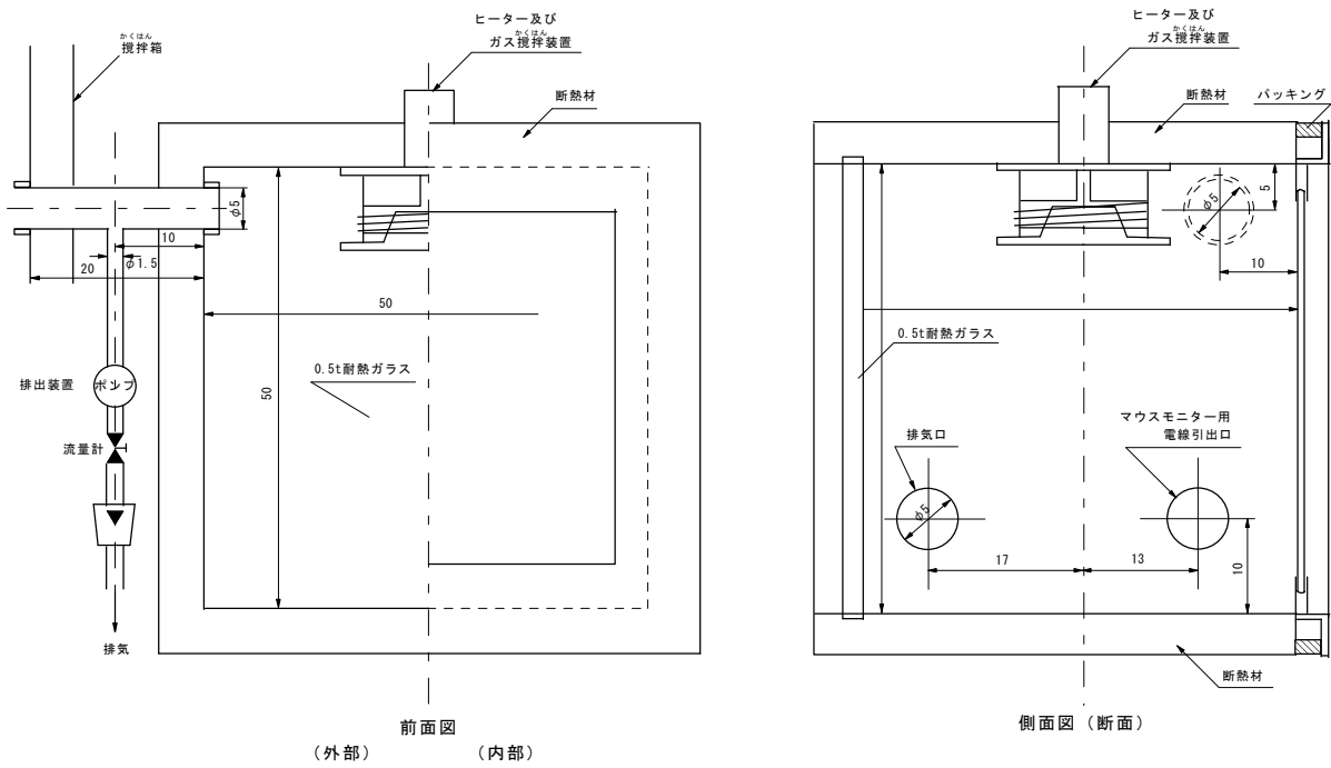
別図8 ガス有害性試験装置の被検箱（寸法単位：cm）（ほ）
