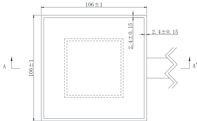
試験体ホルダー(上面図)
