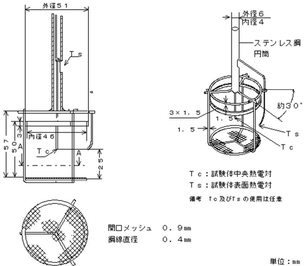
別図2 不燃性試験の試験体ホルダー（寸法単位：mm）（ほ）
