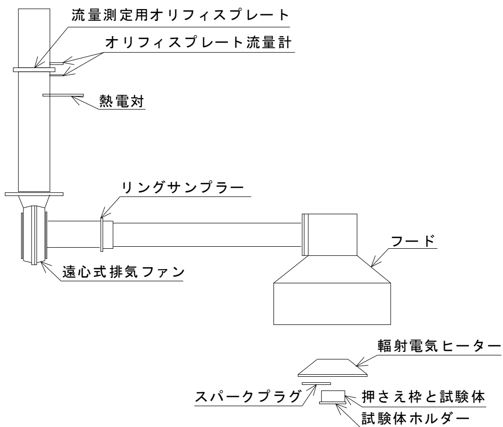
別図3 発熱性試験装置概要(例) (ほ)
