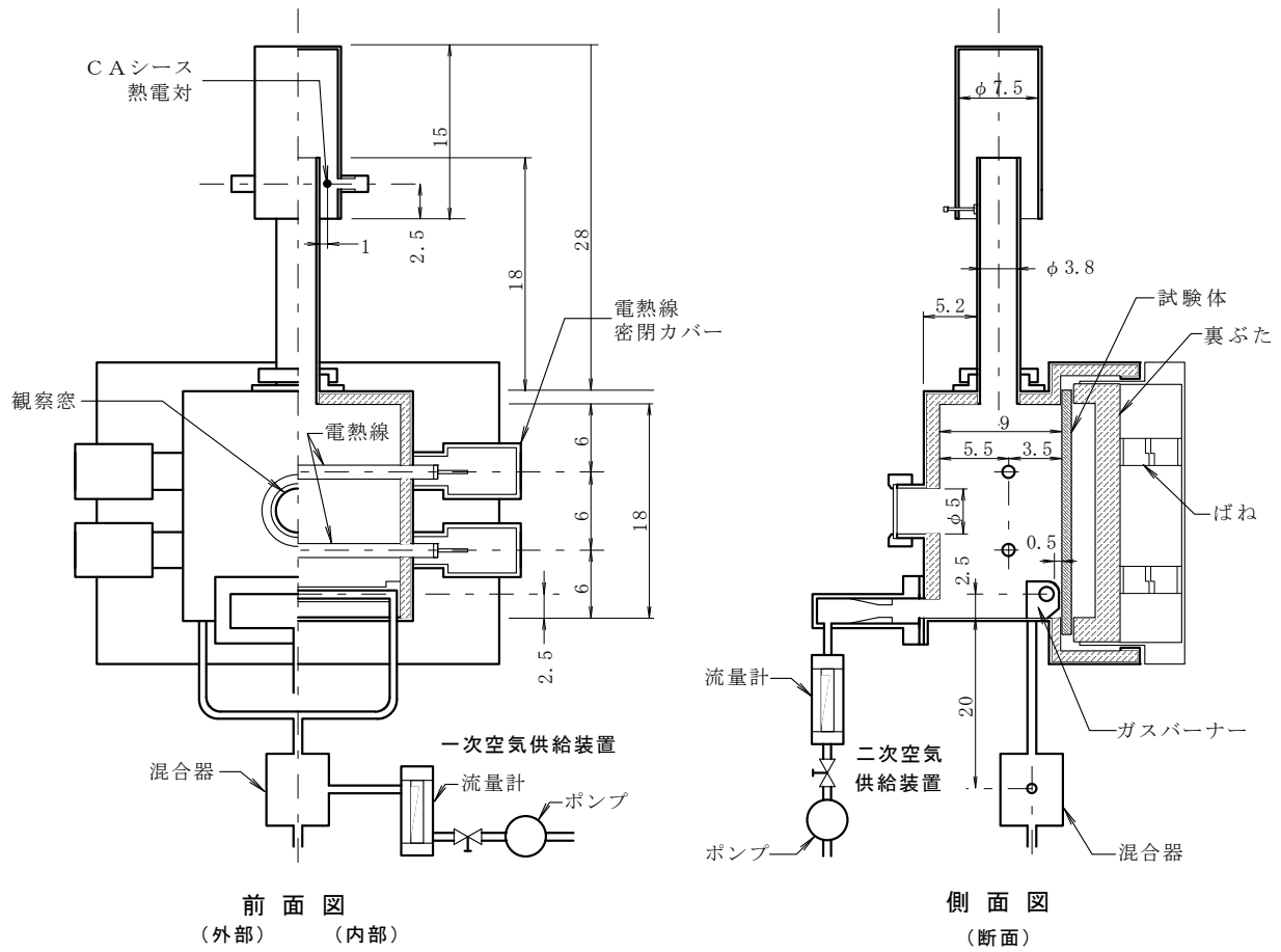
別図6 ガス有害性試験の加熱炉 (寸法単位: cm) (ほ)
