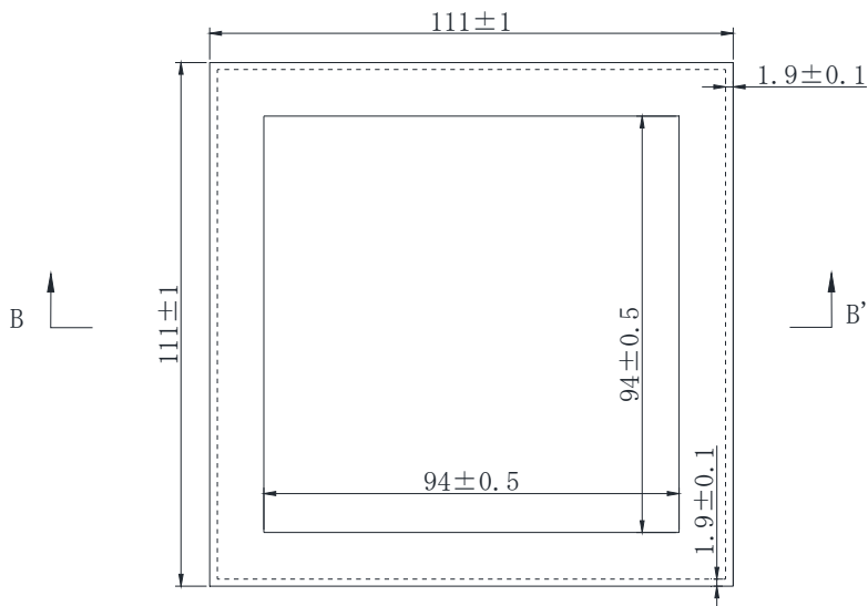
押さえ枠(上面図)
