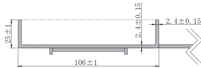
試験体ホルダー(A-A'断面図)
