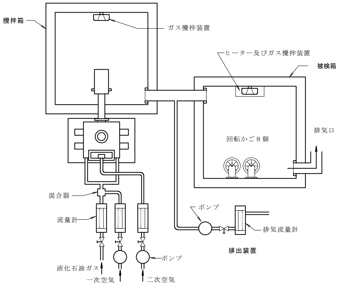
別図5 ガス有害性試験装置 流路図 (ほ)
