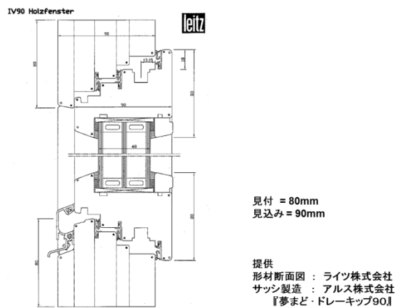
図6 最先端のドレーキップ窓
