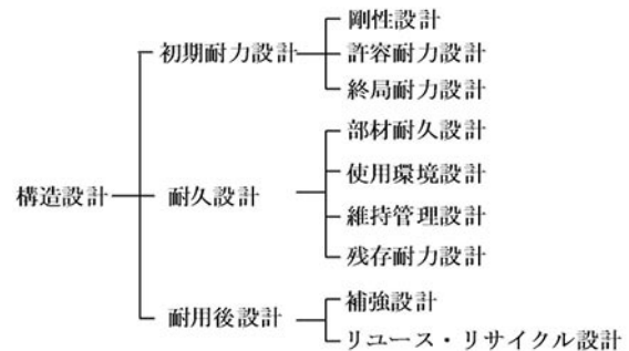
図6 木造住宅の構造設計の項目
