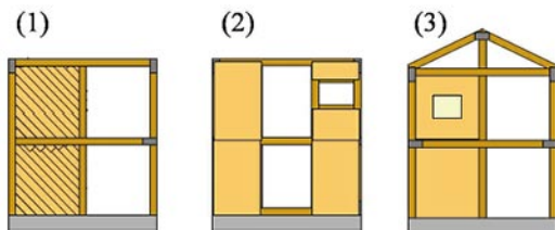
図3 壁式構造
