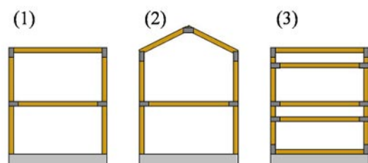
図1 ラーメン構造
