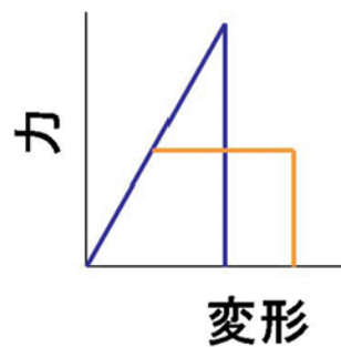
図5 終局限界耐力における力と変形
