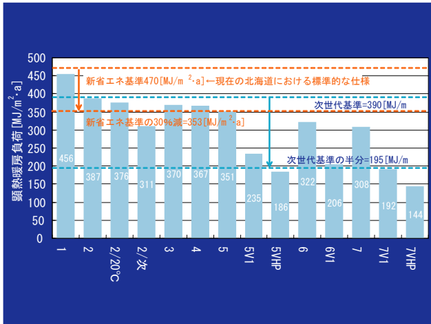
図11 各種仕様と暖房負荷低減
