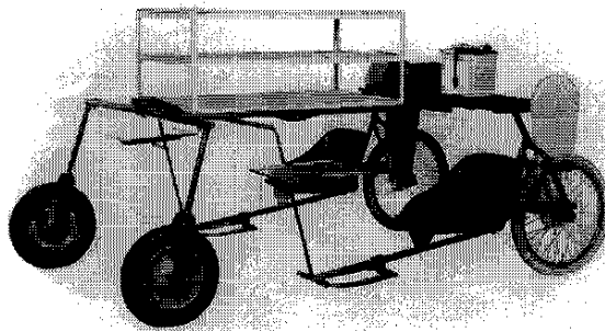
斜視図
