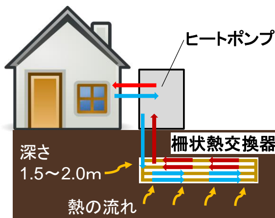
水平採熱式HPシステムの概要
