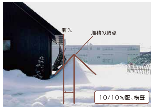
■写真:1 軒下の堆雪状態(上川地方:2月末)
