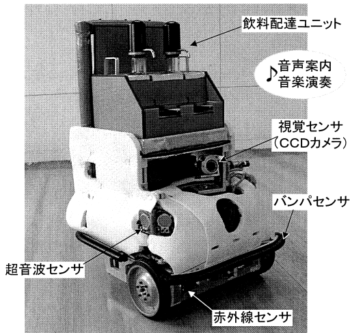
図1 自律型運搬ロボット HIRIX-2
