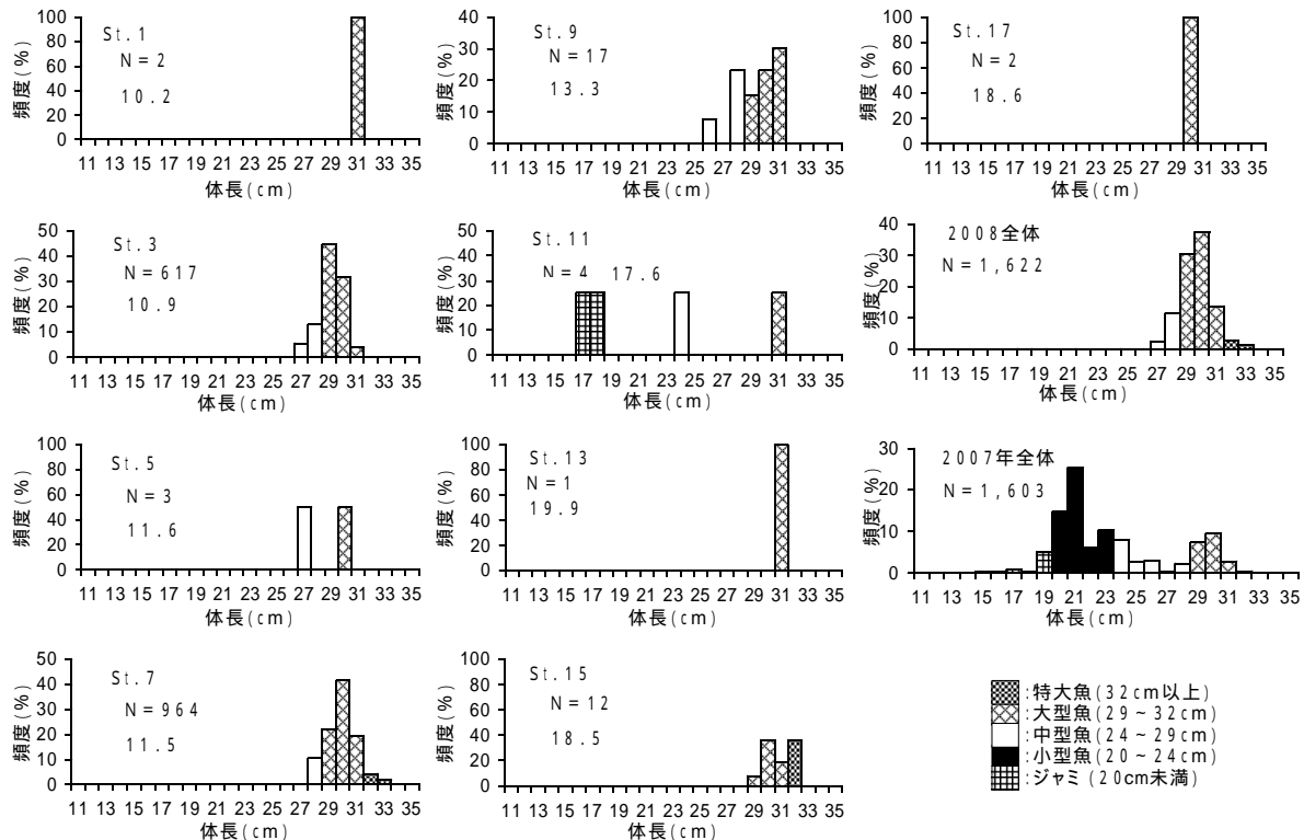
図3 2008年サンマ北上期調査におけるサンマの体長組成 (Nは漁獲尾数)
