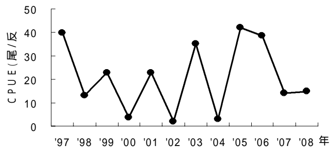
図 2 CPUE の経年変化(目合 : 29,37,48mm)
