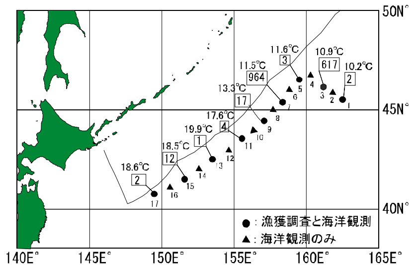
図 1 2008 年サンマ北上期調査点図
