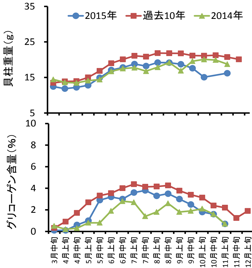
オホーツク南部海域産ホタテガイ貝柱の月旬別性状変化 (2015,2014年および過去10年間(2005~2014年)の平均値)
