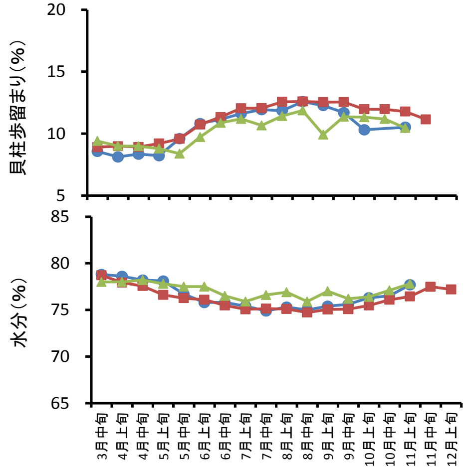
オホーツク南部海域産ホタテガイ貝柱の月旬別性状変化 (2015,2014年および過去10年間(2005~2014年)の平均値)
