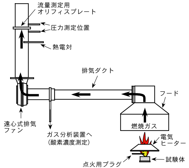
図1 コーンカロリー計装置の概要
