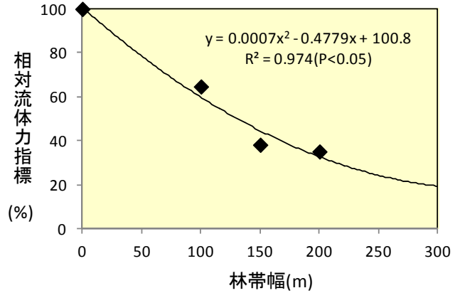
図-2 林帯の拡張が流体力指標に及ぼす効果。相対流体力指標は当該林帯幅の内陸側林縁位置における林帯無しの流体力指標に対する林帯有りの流体力指標の百分率を示す。
