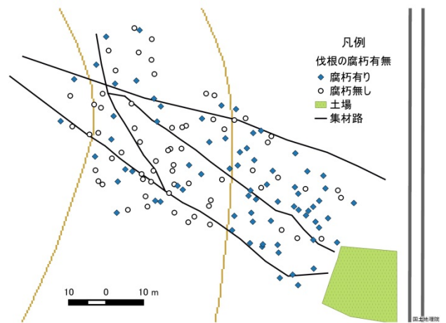
図-1 集材路跡と伐根（腐朽有り・無し）の分布
