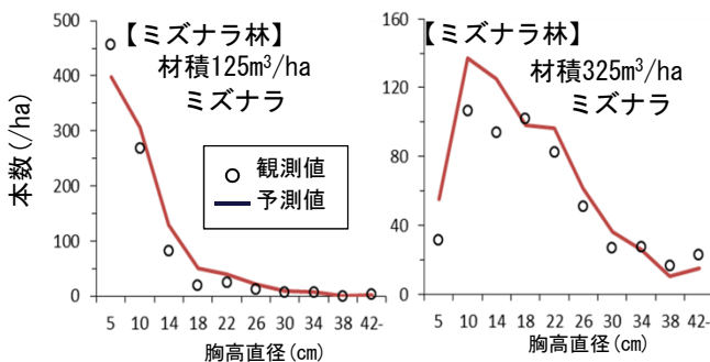
図2 ミズナラ林の森林タイプにおける胸高直径階別の本数 林分材積125m 3 /ha（未成熟林）、325m 3 /ha（成熟林）の条件で胸高直径階ごとの本数をそれぞれ予測した。
