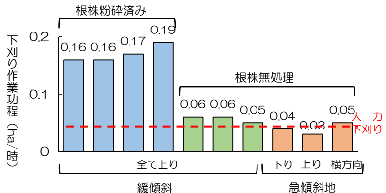
図-1 小型遠隔操縦式草刈機による下刈り作業工期測定結果
