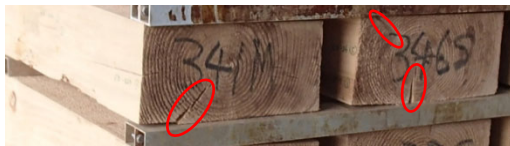
図2 木口からの表面割れ
