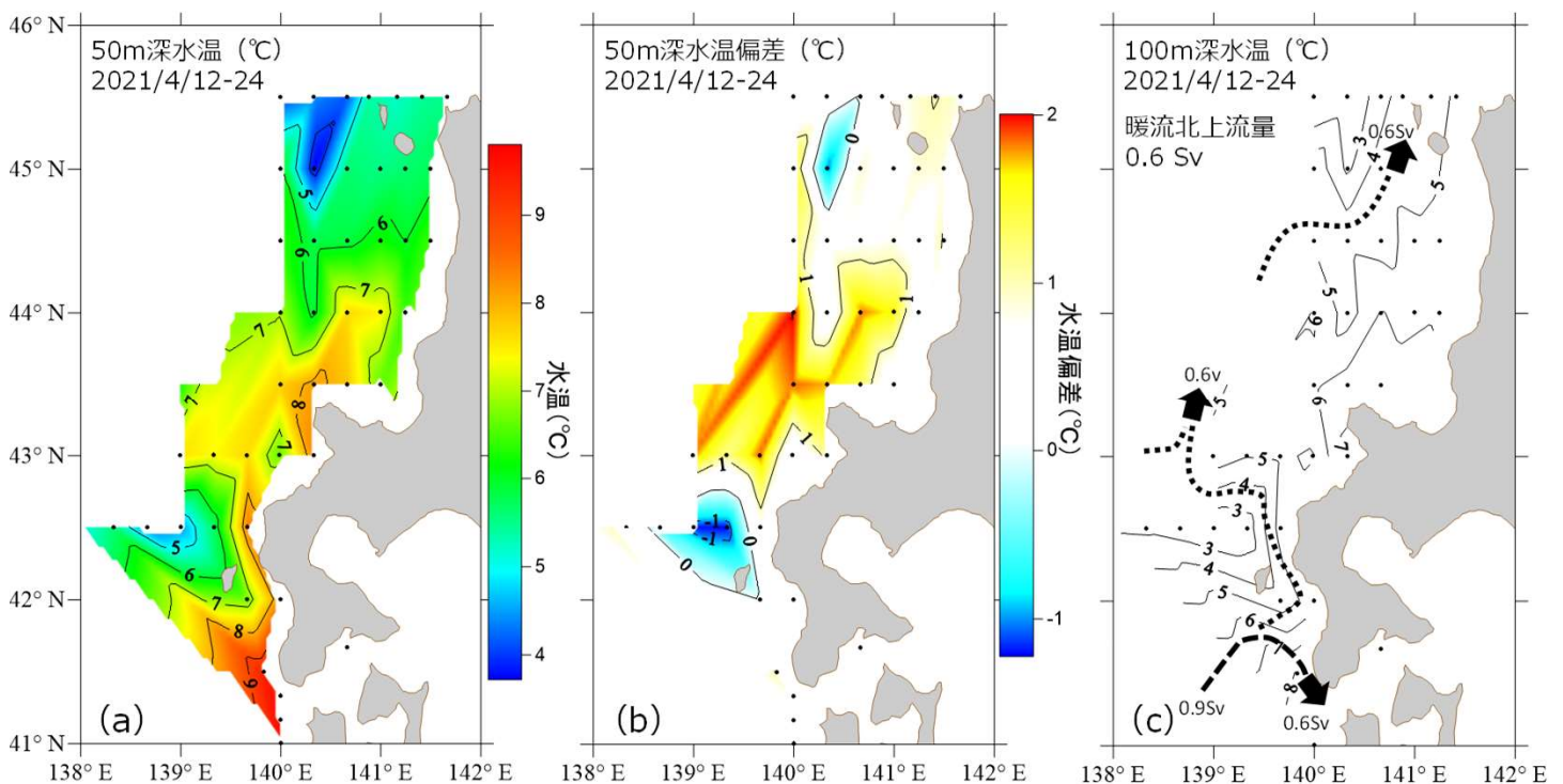
図1 2021年4月中下旬における (a) 50m深水温 (b) 50m深水温偏差の水平分布、(c) 100m深水温の水平分布と対馬暖流の流路。水温偏差は過去30年（1989年～2018年）の平均値から算出。流量の単位はSv（=1×10 6 m 3 /s）。
