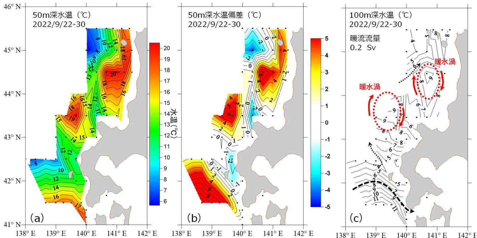
図1 2022年9月下旬における (a) 50m深水温 (b) 50m深水温偏差の水平分布、(c) 100m深水温の水平分布と対馬暖流の流路(矢印)。水温偏差は過去30年(1989年～2018年)の平均値から算出。流量の単位はSv (=1×10 6 m 3 /s)。
