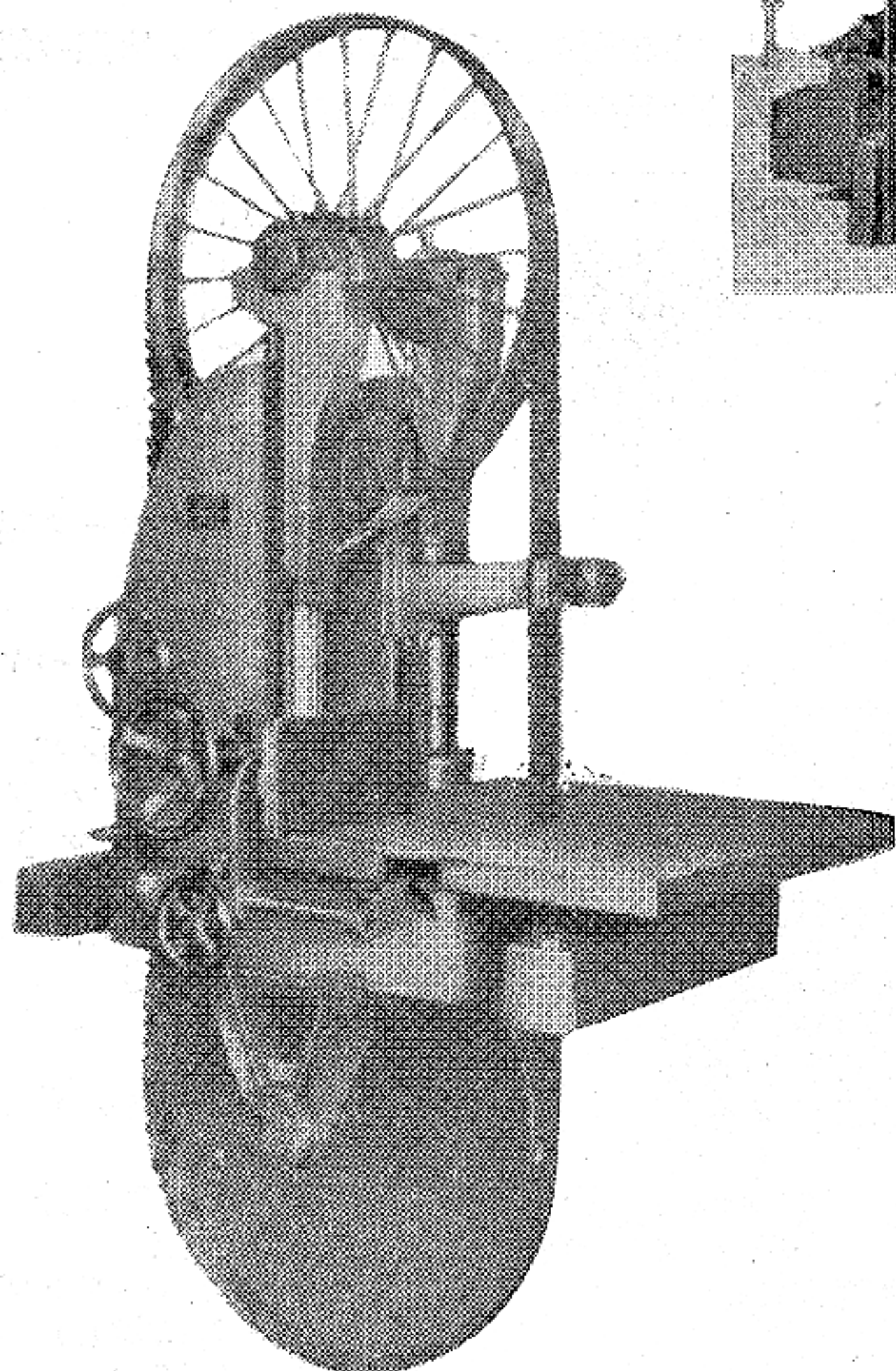
42" 高速度テーブルバンドソー
