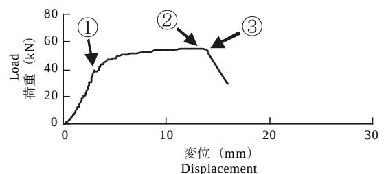
第4図 荷重 - 変位曲線(割れが影響した場合)
