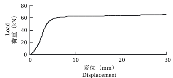
第3図 荷重 - 変位曲線(割れの影響が小さい場合)
