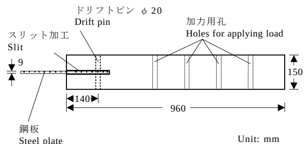
第1図 試験体 Fig. 1. Specimen.
