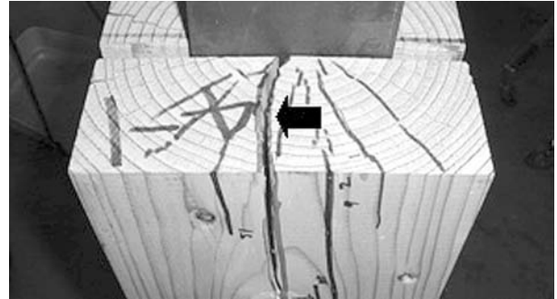
第7図 破壊の進行状況（終局時）
