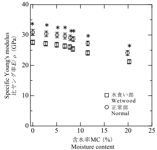
第4図 含水率に対する比ヤング率の変化
