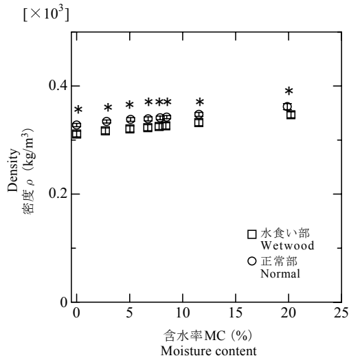
第2図 含水率に対する密度の変化
