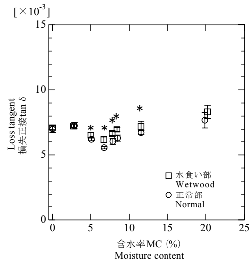
第5図 含水率に対する損失正接の変化
