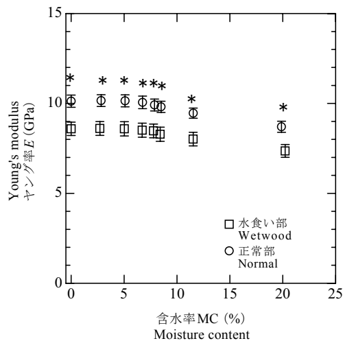
第3図 含水率に対するヤング率の変化
