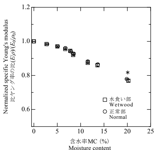
第6図 比ヤング率の比
