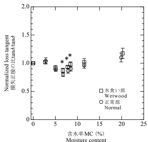
第7図 損失正接の比
