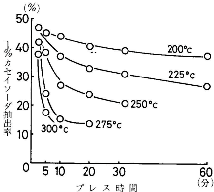
第7図 プレス条件と1%カセイソーダ抽出率・HCl・HCHO ppt の関係
