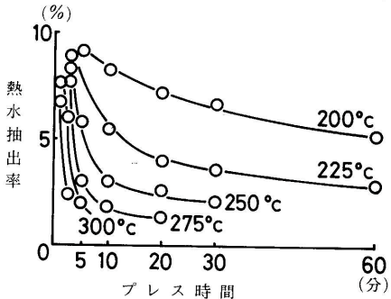
第6図 プレス条件と熱水抽出率・HCl・HCHO ppt の関係
