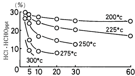
第6図 プレス条件と熱水抽出率・HCl・HCHO ppt の関係
