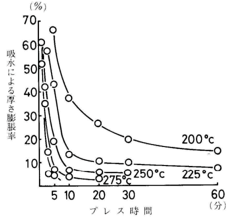
第2図 プレス条件と吸水による厚さ膨張率の関係
