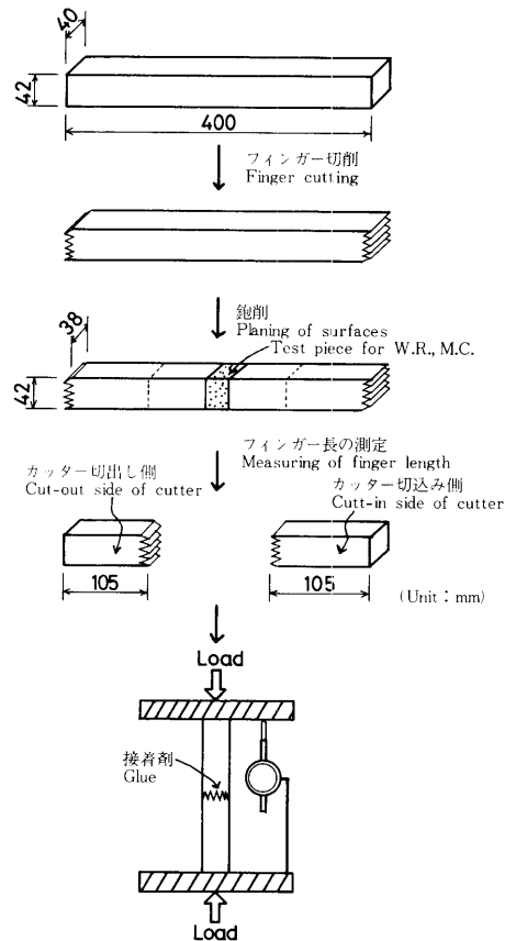
第14図 小断面材による嵌合縦圧縮試験の手順 Fig. 14 Preparation of small specimens and method for inserting test .
