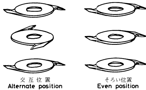
第6図 隣接カッターの刃先位置 (因子A) Fig.6 Position of knife edge of cutter (Factor A).
