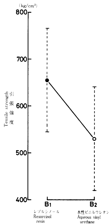
第21図 接着剤 (因子B) の効果グラフ Fig. 21 Effect graph of glue (Factor B).
