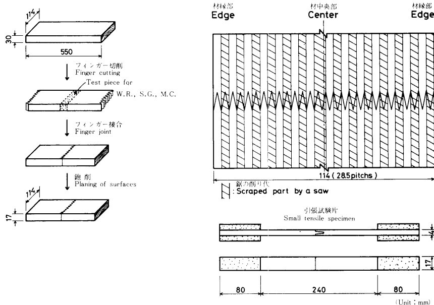
第19図 フィンガージョイント材の製造手順と引張試験片の木取方法
