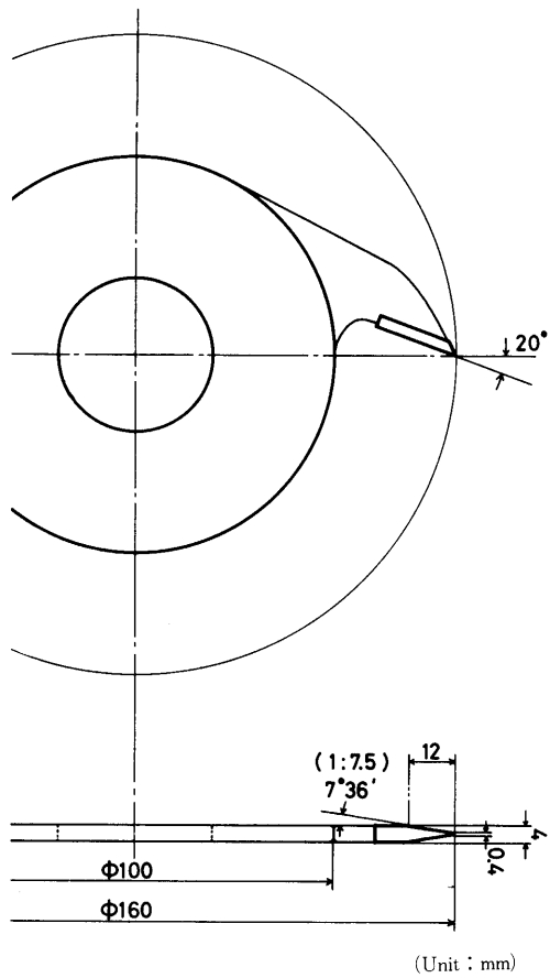
第5図 本報告で使用したカッターの公称寸法 Fig.5 Nominal size of mini-finger cutter used in this report.
