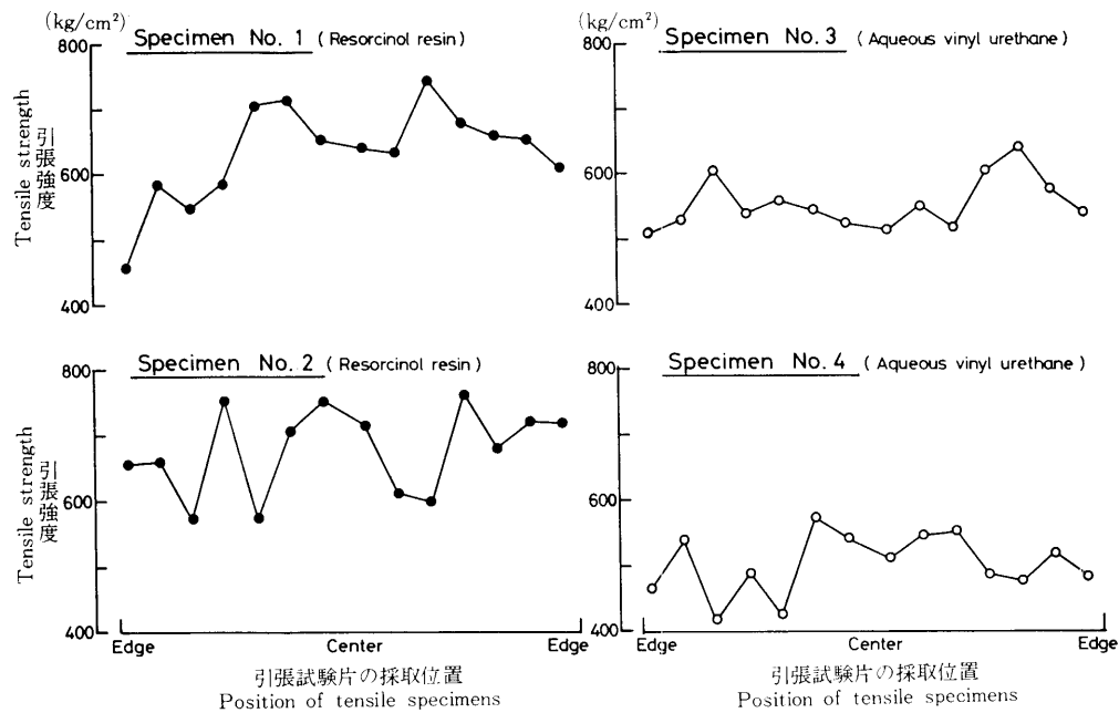
第20図 引張試験片の採取位置と引張強度の関係 Fig. 20 Relationship between tensile strength and position of tensile specimen.
