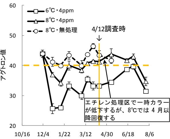
図 1 エチレン処理および貯蔵温度がチップカラーに及ぼす影響（スノーデン、2009年産） 士幌町内の異なる4生産者の平均値。 アグトロン値：ポテトチップスの色を表す指標。値が大きい方が望ましく、本成績では40以上で原料として使用可能とした。
