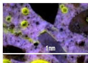
コンクリート中の微細なひび割れ
