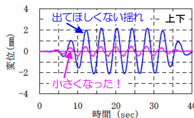
①の制御効果の一例
