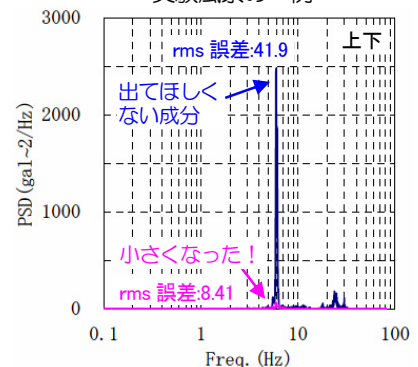
②の制御効果の一例
