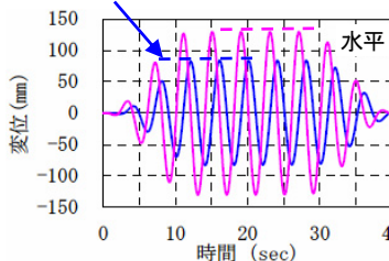
①の制御効果の一例
