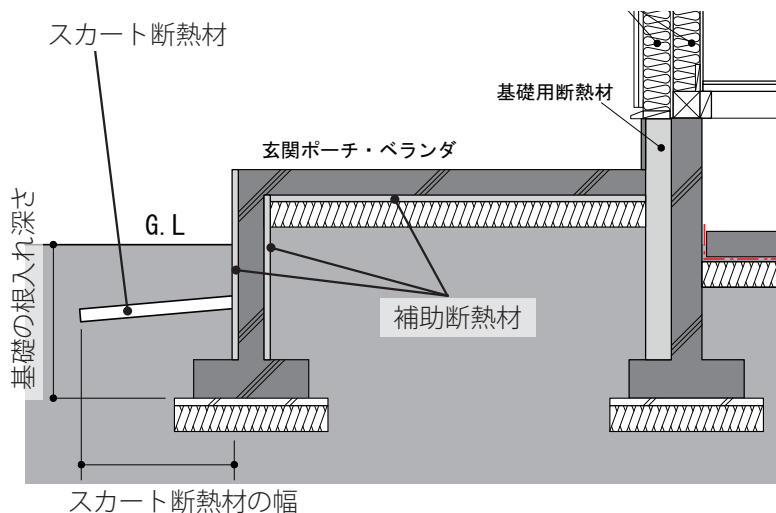
図 3-4 各断熱材の名称と幅、深さの定義
