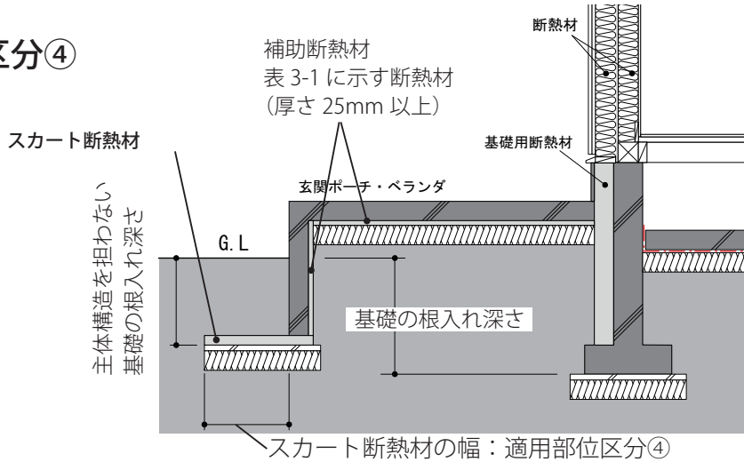
図 3-9 ポーチ等部の主体構造を担わない基礎の根入れ深さ及び断熱材幅①
