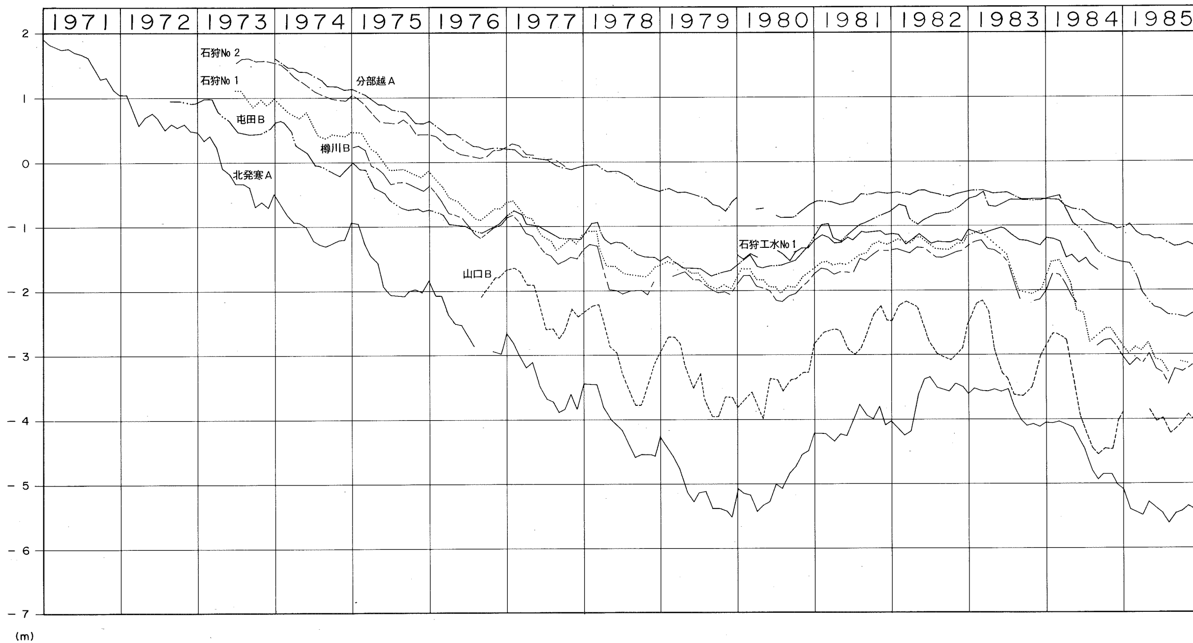
観測井水位経年変化図(c)
