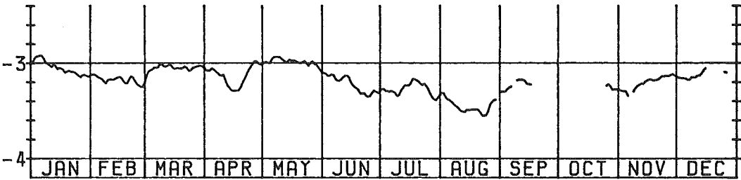
樽川観測所 B水位 深度 200m
