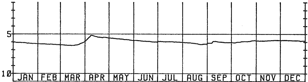
樽川観測所 A沈下
