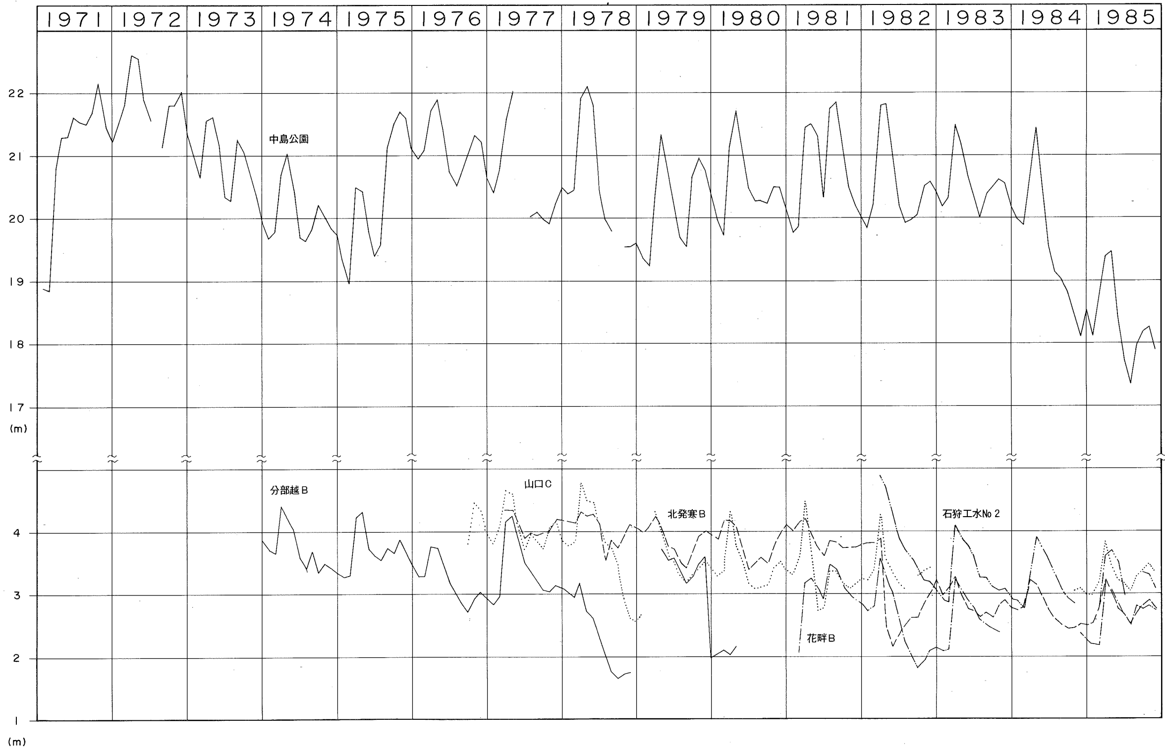
観測井水位経年変化図(A)
