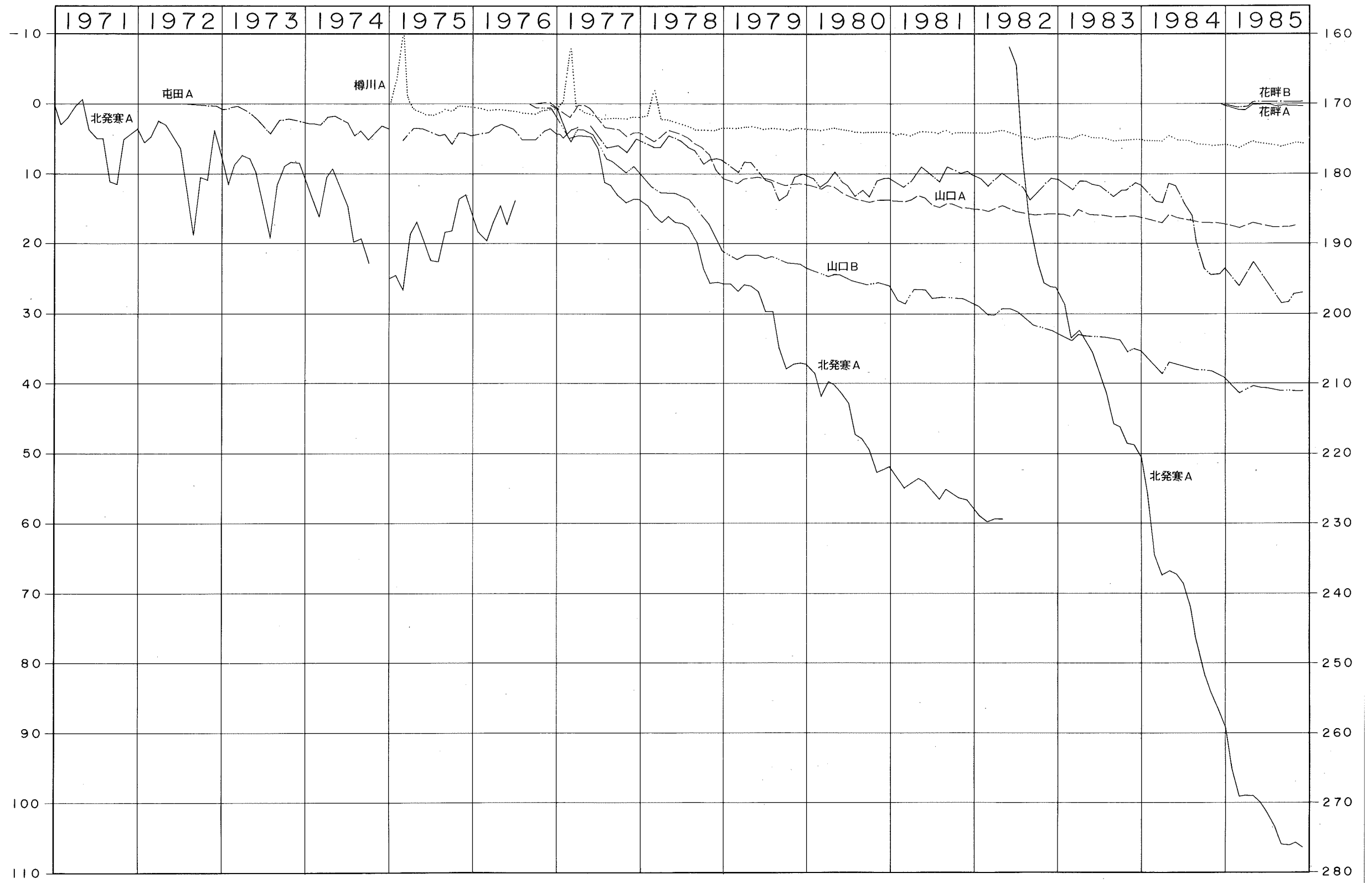
観測井地盤沈下経年変化図
