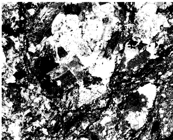
第11図 酸性脈岩（岩松ダム付近）
