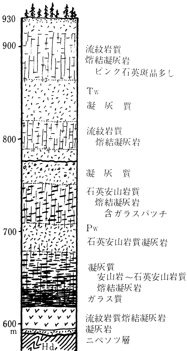
第3図 パンケニコロ 熔結凝灰岩，十勝熔結凝灰岩柱 状断面 (パンケニコロ川上流)
