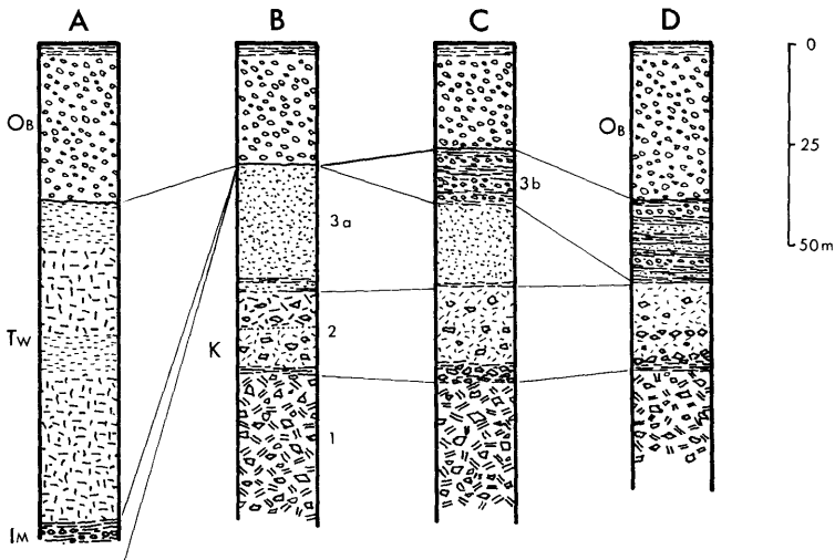
第2図 美蔓台地における屈足層の柱状断面図
