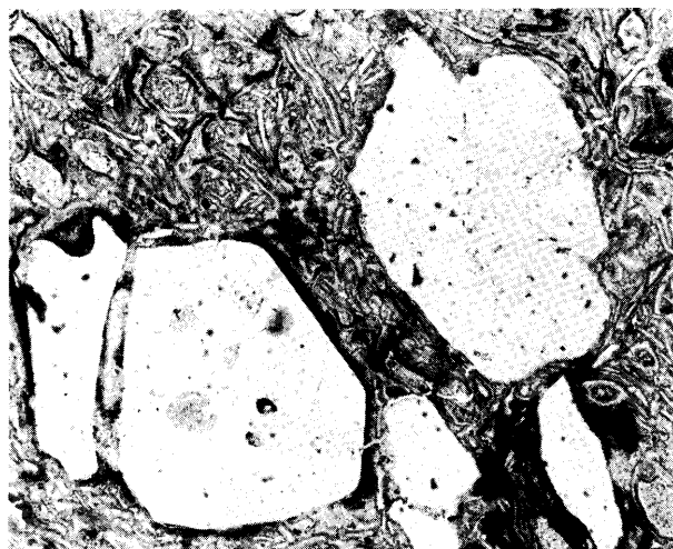
第1図 流紋岩質熔結凝灰岩
