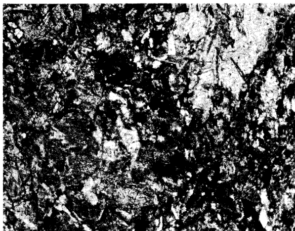
第13図 輝 緑 岩 (オソウシ川)
