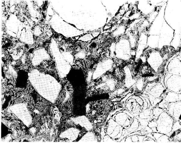
第7図 十勝熔結凝灰岩 大形石英斑晶，破片状の斜長石，石英，板状 黒雲母，ガラス（パーライト状）のパッチ
