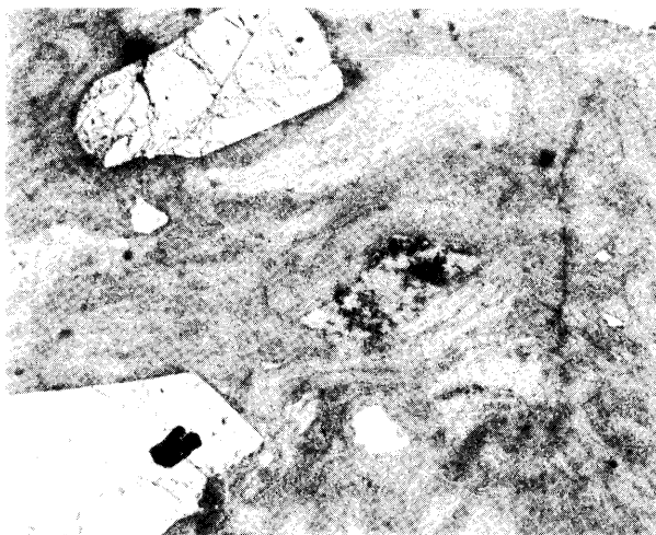
第4図 パンケニコロ熔結凝灰岩 下底部の流紋岩質部。有色鉱物はない。
