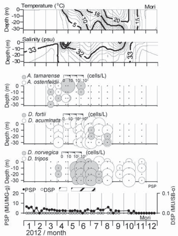
図2-4 森調査地点における水温と塩分の季節変化、 Alexandrium 属2種と Dinophysis 属4種の出現状況と漁獲対象二枚貝（ホタテガイ）の毒性値の推移（PSP:麻痺性貝毒, DSP:下痢性貝毒）と出荷規制状況（斜線は自粛規制期間, 網目は自主規制期間）
