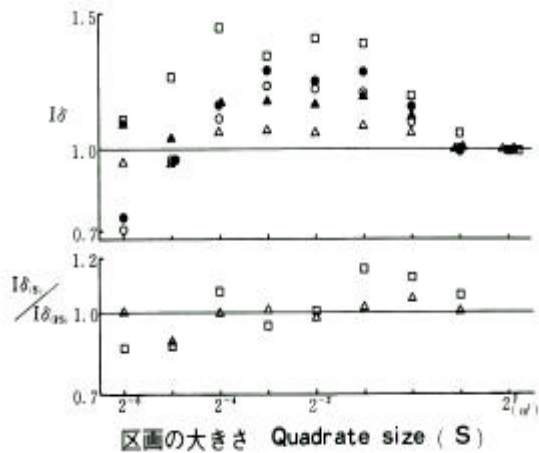
図-11 I δ -値、I δ s /I δ 2s と区画の大きさとの関係
