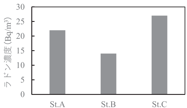
図3 上ノ国漁港底層水のラドン濃度
