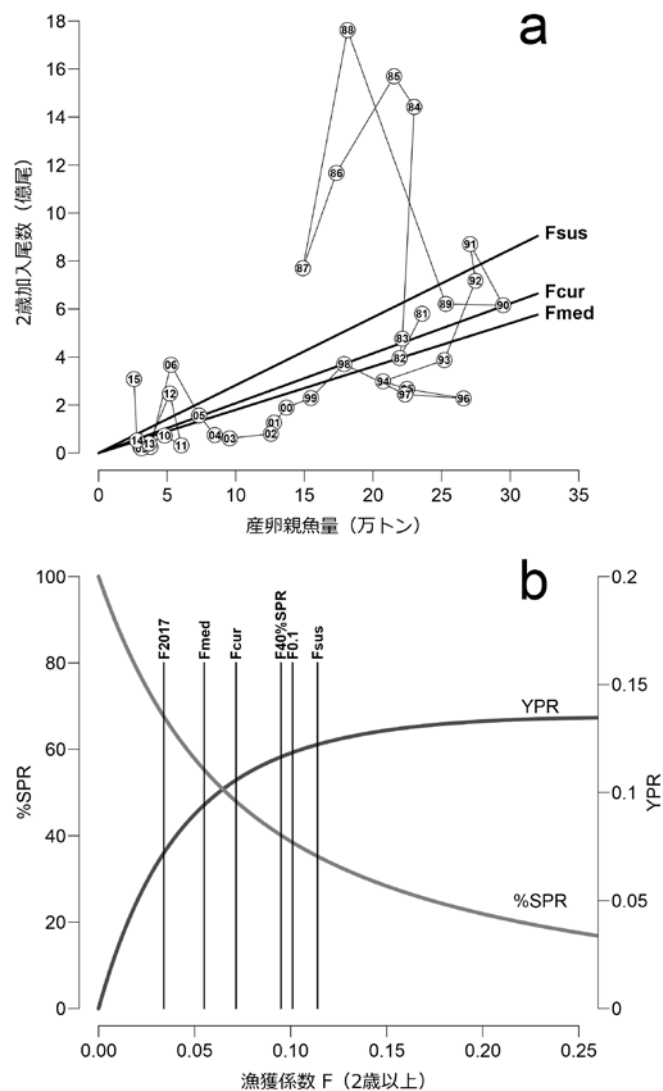
図 10 F_{cur} , F_{2017} と管理基準値 ( F_{sus} , F_{med} , F_{40\%SPR} , F_{0.1} ) の比較
