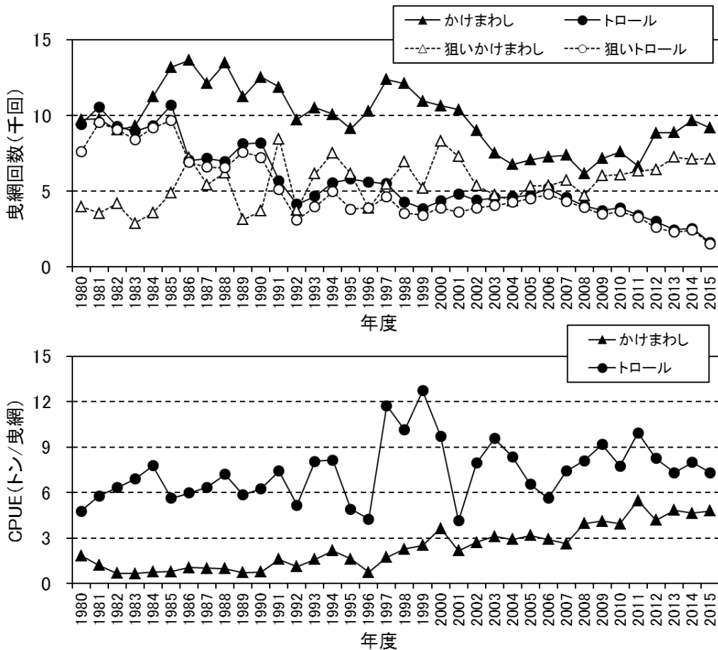
図3 道東太平洋における沖合底びき網漁業によるスケトウダラの 曳網回数(上), CPUE(下)の経年変化 (資料：北海道沖合底びき網漁業漁場別漁獲統計)
