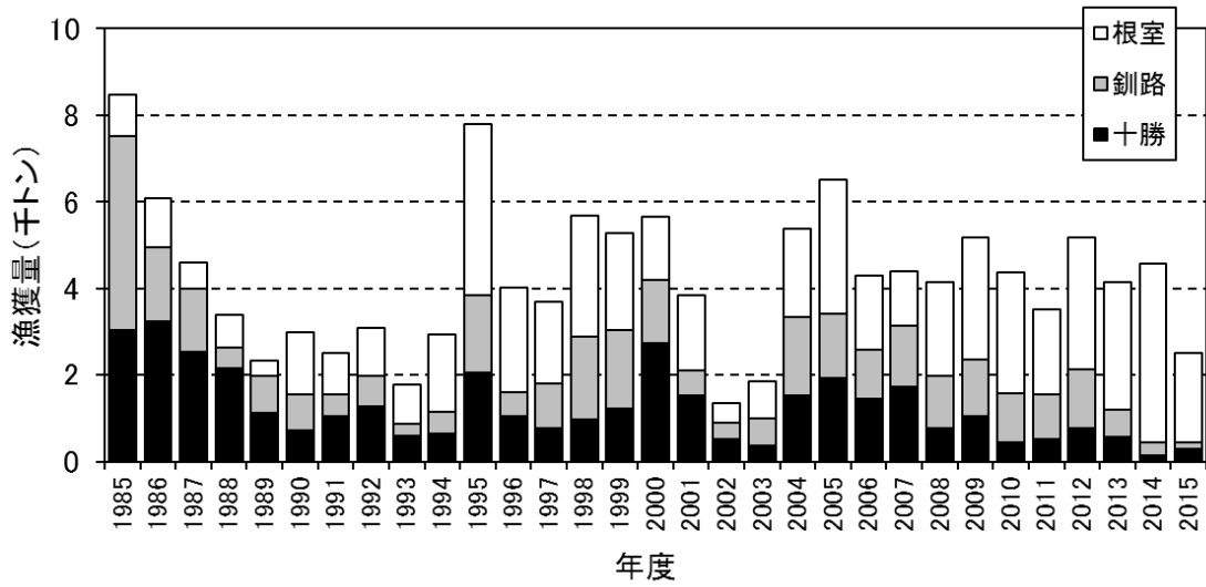
図2 道東太平洋における沿岸漁業によるスケトウダラ漁獲量の経年変化 (資料：漁業生産高報告, 2014, 2015年度は水試集計速報値)
