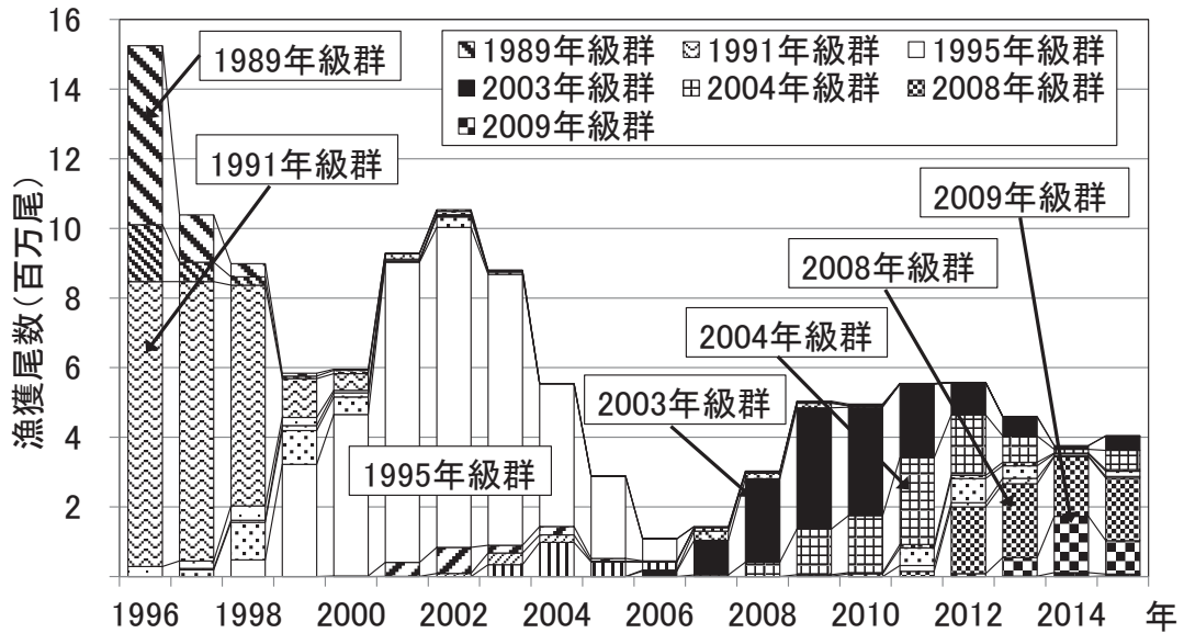
図5 噴火湾海域におけるアカガレイの年級群別漁獲尾数
