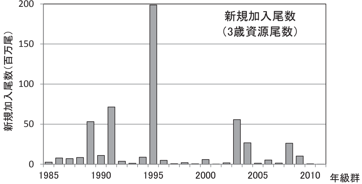
図7 アカガレイ3歳魚の資源尾数の推移
