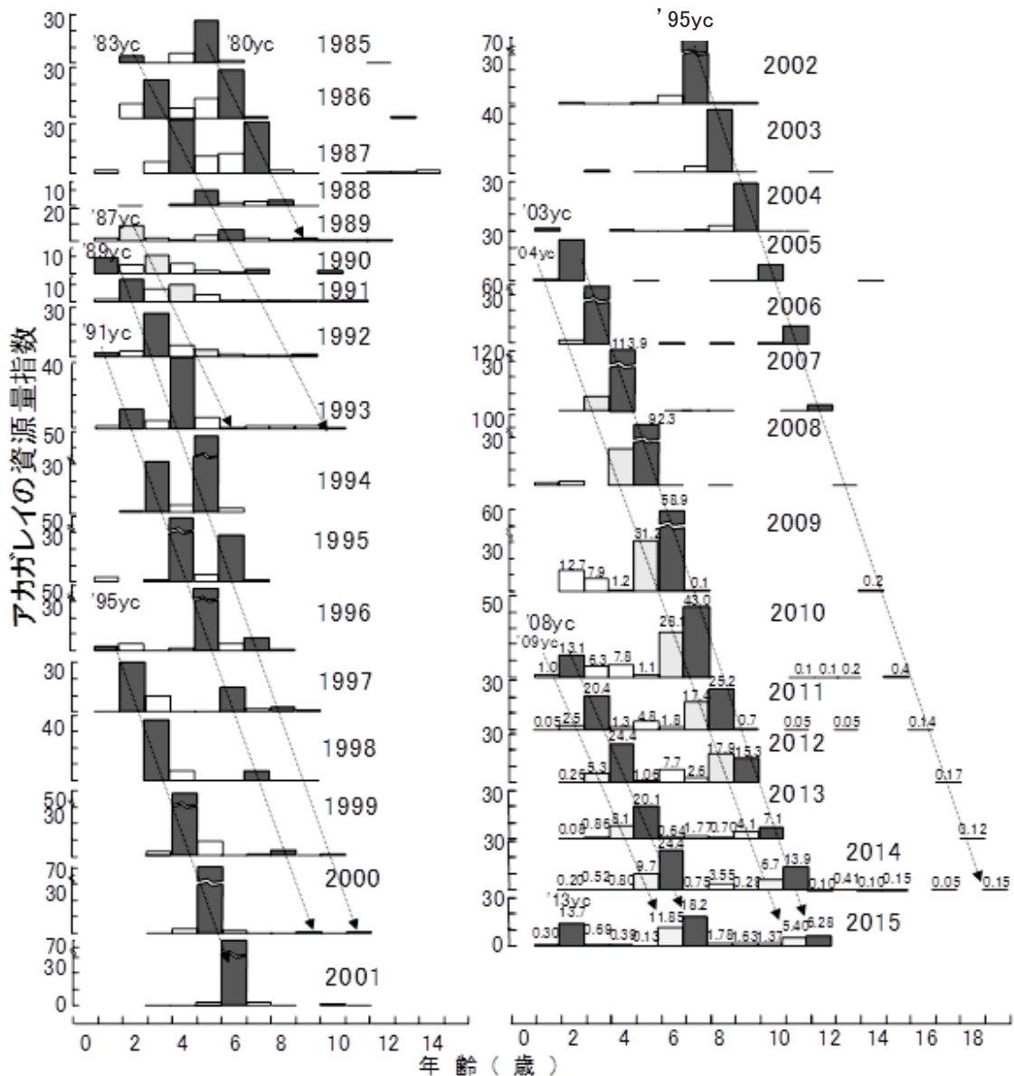
図6 北大うしお丸の着底トロール網によって漁獲されたアカガレイの年級群別相対資源量指数の経年変化(高津ら 1) より)
