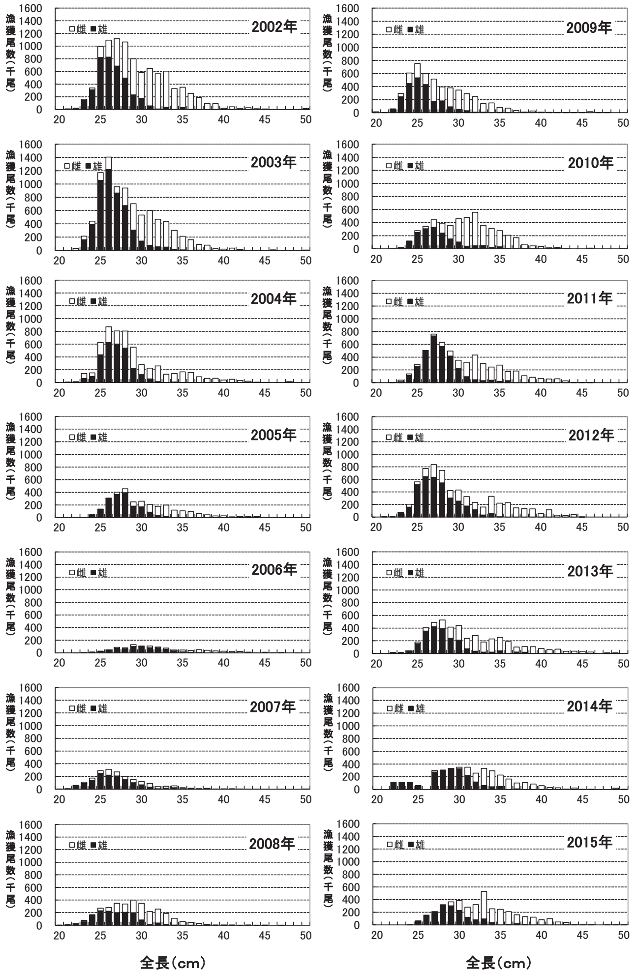
図4 アカガレイ刺し網漁獲物の全長組成の経年変化
