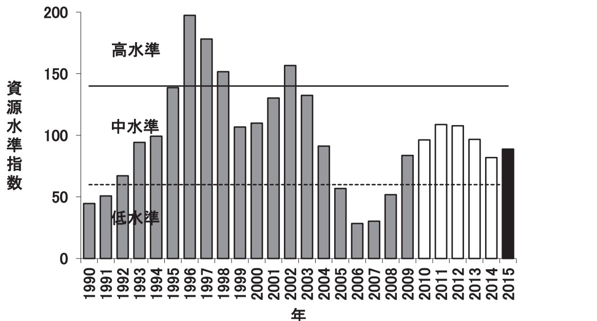
図11 噴火湾海域におけるアカガレイの資源水準(資源状態を示す指標:漁獲量)
