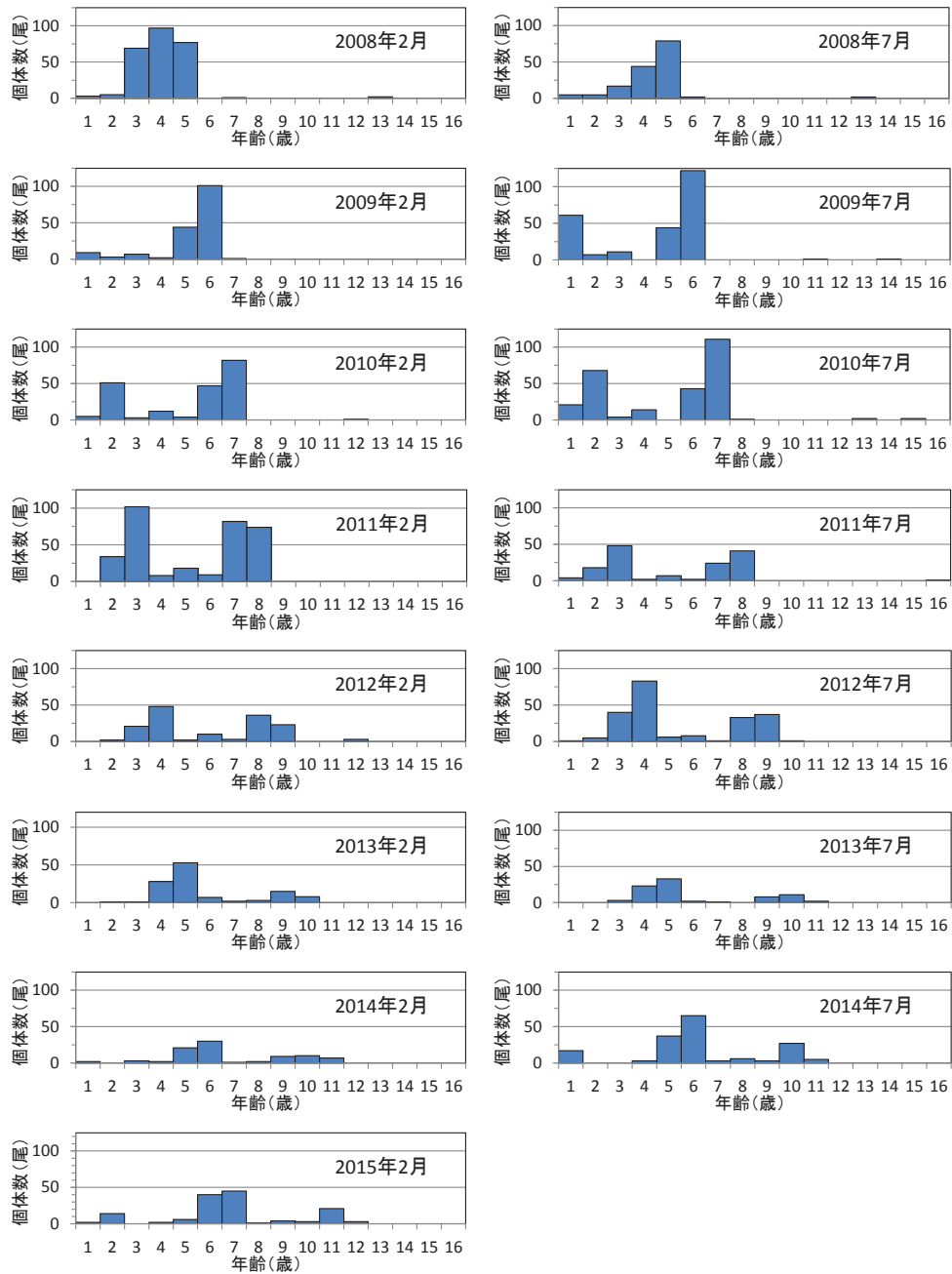
図10 函館水産試験場によるソリネット調査で採集されたアカガレイの年齢組成
