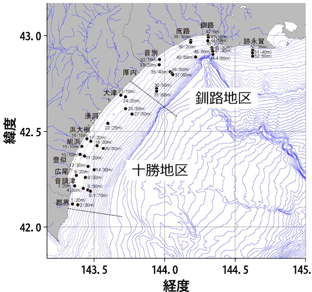
図4 調査CPUEの算出に用いた十勝・釧路海域漁期前調査の調査点 (数字は調査点番号, 括弧内は水深)
