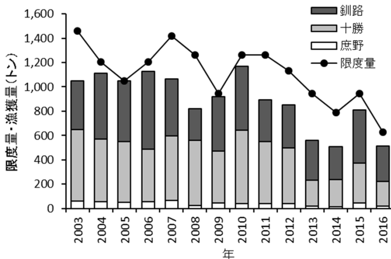
図2 ししゃもこぎ網漁業の「目安の漁獲限度量」と実績漁獲量の推移 (単位:トン)
