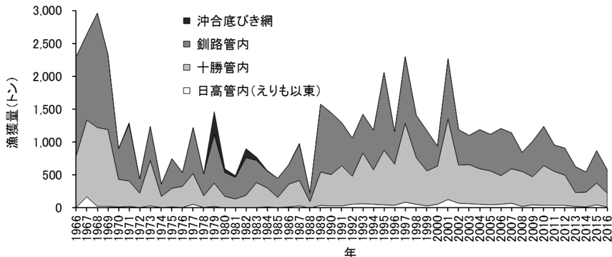
図1 沿岸漁業(庶野, 十勝, 釧路海域)および沖合底びき網漁業におけるシシャモ漁獲量の経年変化(単位:トン) (2003年以降, 限度量制が導入された)
