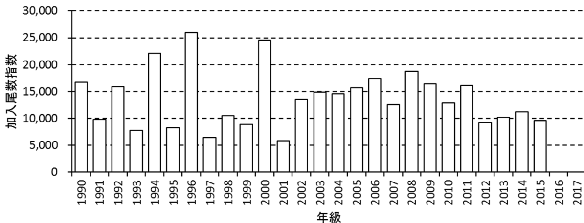
図8 加入尾数指数の経年変化
