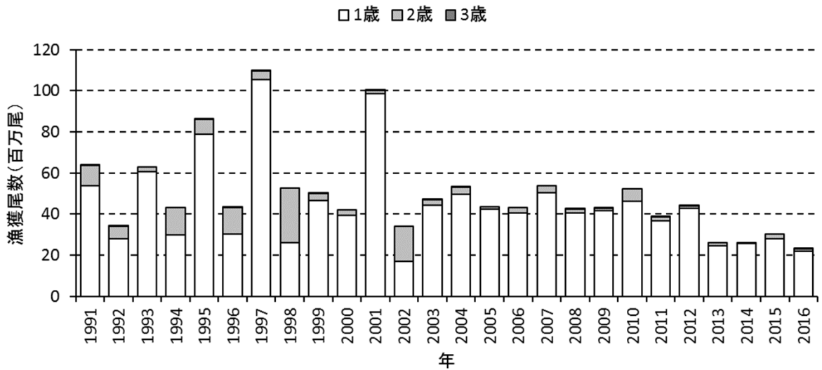
図7 十勝・釧路海域におけるししゃもこぎ網漁業による年齢別漁獲尾数の経年変化
