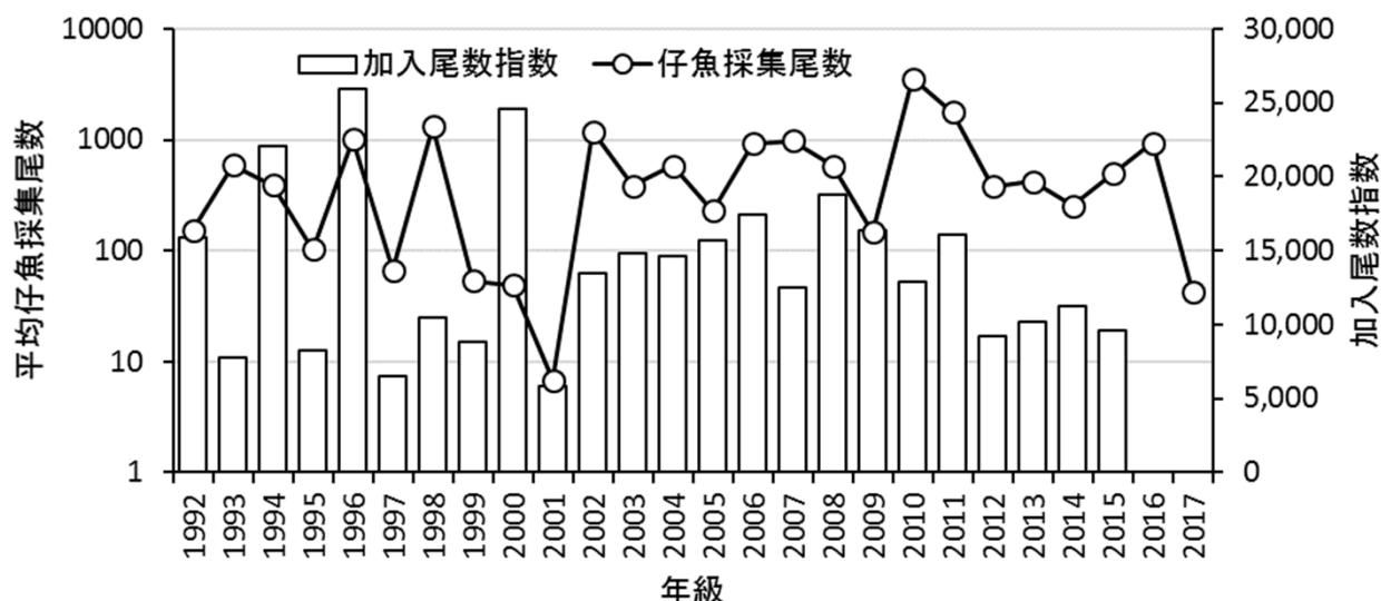
図12 新釧路川において実施した降海仔魚調査による平均仔魚採集尾数と加入尾数指数の推移
