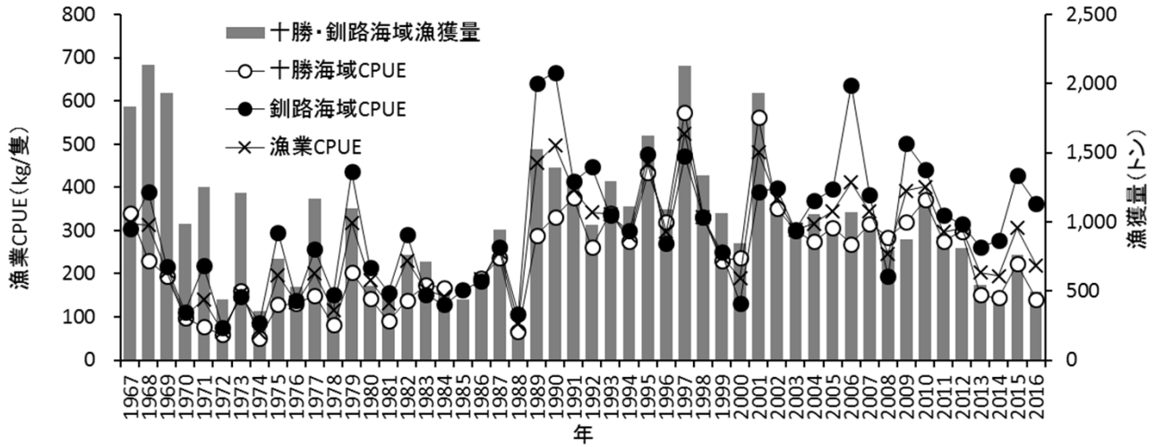
図6 十勝, 釧路海域におけるししゃもこぎ網漁業の漁獲量とCPUE(漁業CPUE)の経年変化
