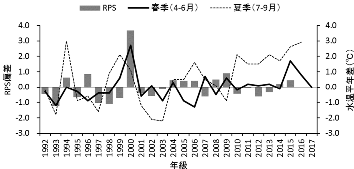
図13 釧路沖の海面水温偏差とRPS偏差の推移
