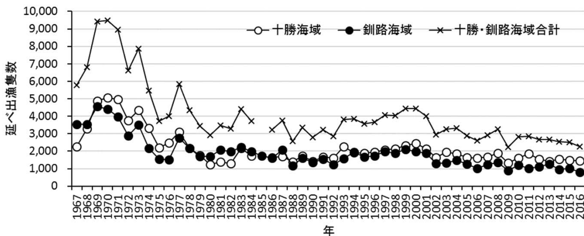
図3 十勝, 釧路海域におけるししゃもこぎ網漁業の延べ出漁隻数(隻)の経年変化
