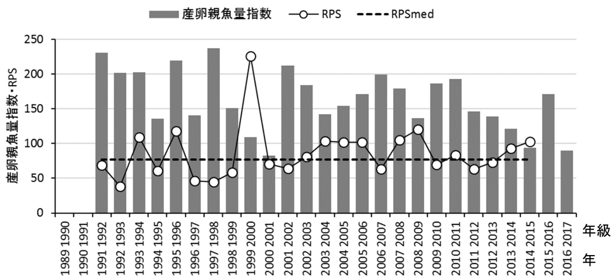
図9 産卵親魚量指数とRPSの経年変化 (横軸の年級および年は、RPSおよび産卵親魚量指数にそれぞれ対応する)
