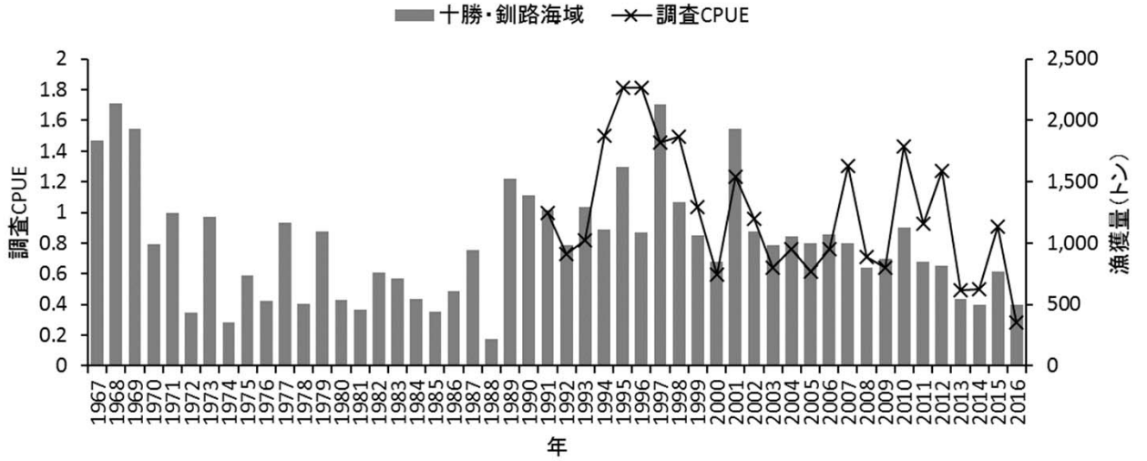
図5 十勝・釧路海域における漁期前調査の漁獲量と標準化CPUE(調査CPUE)の推移
