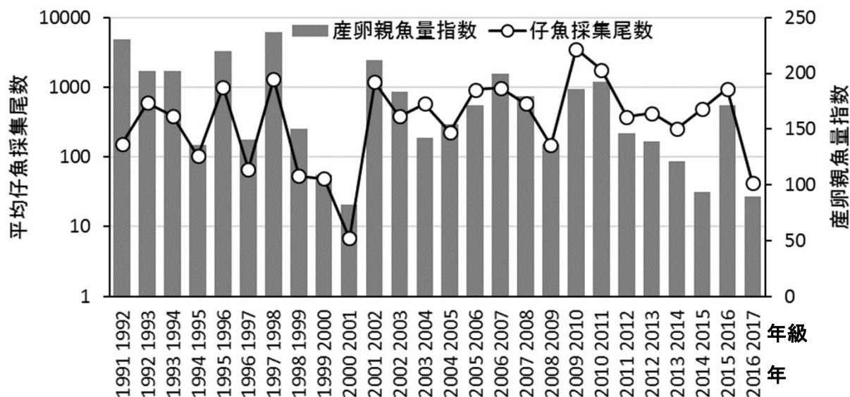
図11 新釧路川において実施した降海仔魚調査による平均仔魚採集尾数と産卵親魚量指数の推移 (横軸の年級および年は、RPSおよび産卵親魚量指数にそれぞれ対応する)
