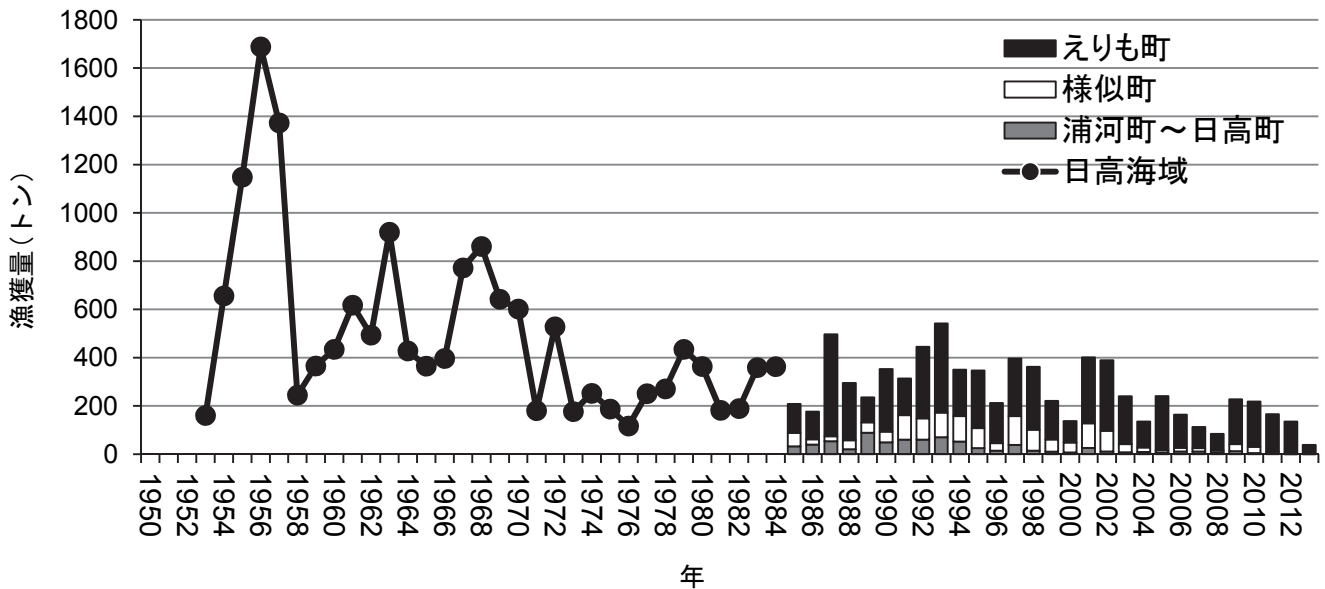
図3 日高海域におけるハタハタ漁獲量の推移
