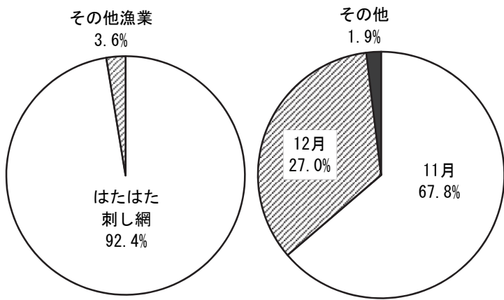
図1 日高海域におけるハタハタの漁業種別（左）および月別（右）の漁獲量比率（2009～2013年の平均値）
