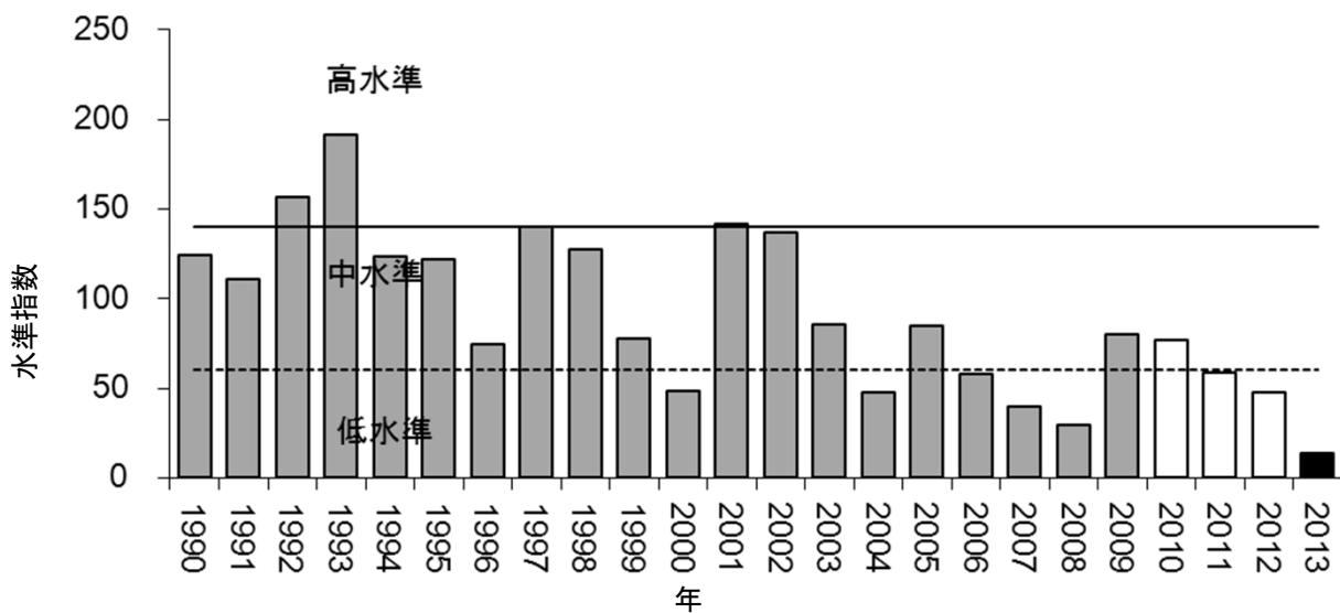
図8 日高海域におけるハタハタの水準指数(グラフ内のデータは漁獲量) グレーは基準年、黒は評価年を示す。
