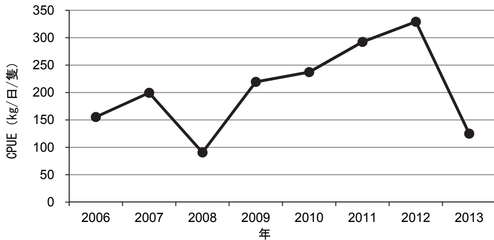
図6 えりも漁協におけるはたはた刺し網漁業のCPUEの推移
