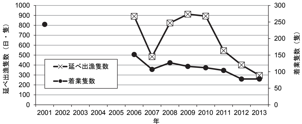
図4 えりも漁協におけるはたはた刺し網漁業の延べ出漁隻数（日・隻）および着業隻数（隻）の推移
