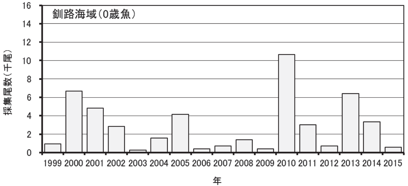
図9 魚群分布調査(釧路海域9~10月)におけるハタハタ0歳魚採集尾数の経年変化
