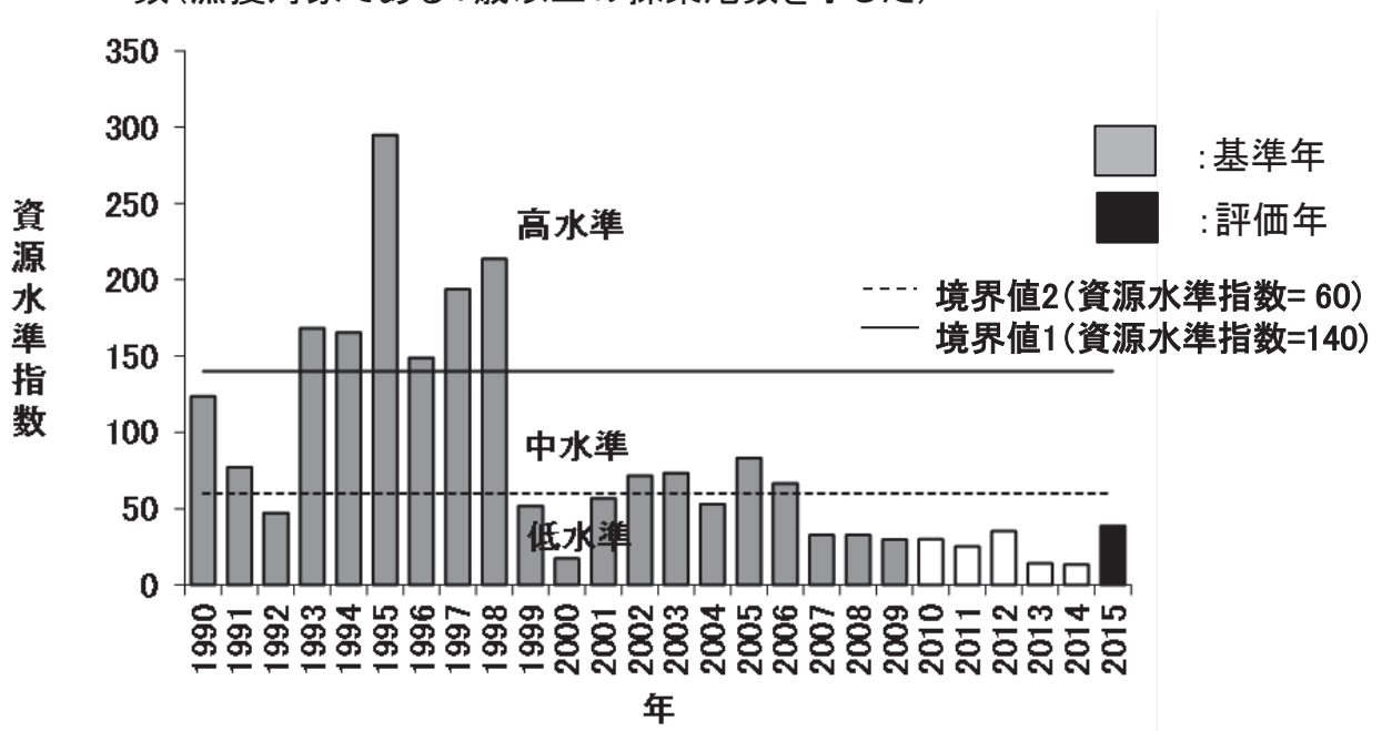
図8 道東太平洋海域におけるハタハタの資源水準 資源状態を示す指標：9~12月の釧路沿岸および根室沿岸の漁獲量)
