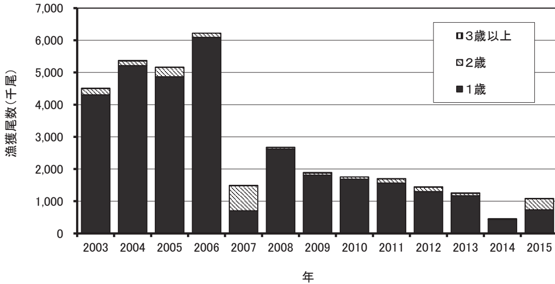
図6 釧路海域沿岸漁業における推定年齢別漁獲尾数(9~12月)の経年変化
