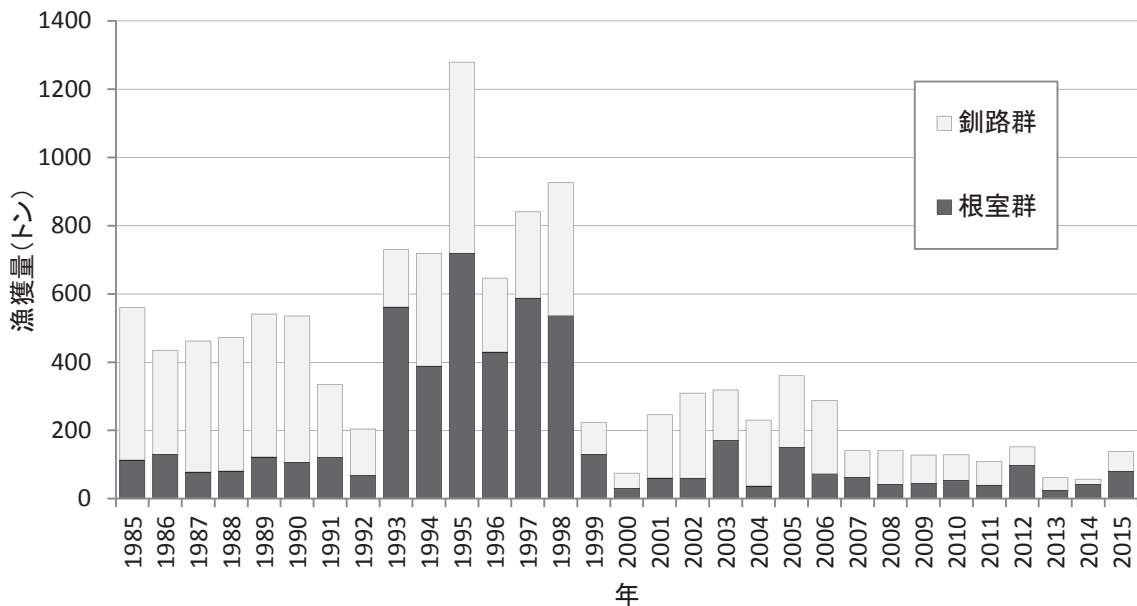
図5 釧路群および根室群における産卵親魚の漁獲量(9~12月の釧路海域および根室海域における沿岸漁業の漁獲量)
