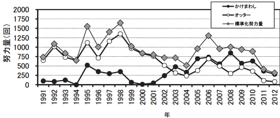
図4 イカナゴ専獲(80%以上)条件により抽出された努力量および標準化された努力量の推移
