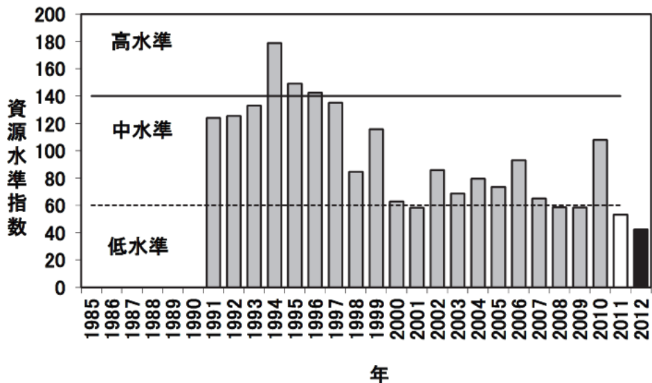
図8 宗谷海峡海域のイカナゴ類の資源水準 (資源状態を示す指標:標準化 CPUE) (基準年を1991年から2010年までの20年間とした)
