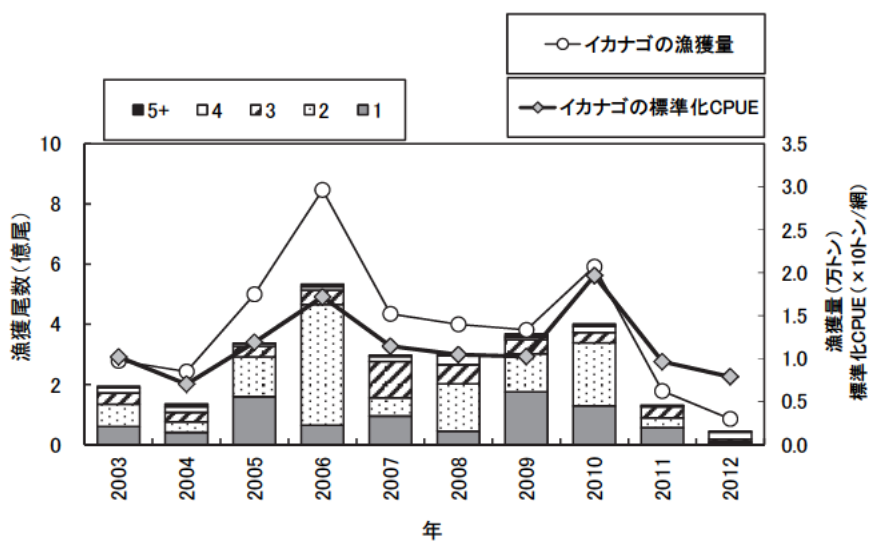
図 6 イカナゴの年齢別漁獲尾数, イカナゴのみの漁獲量および標準化 CPUE の推移
