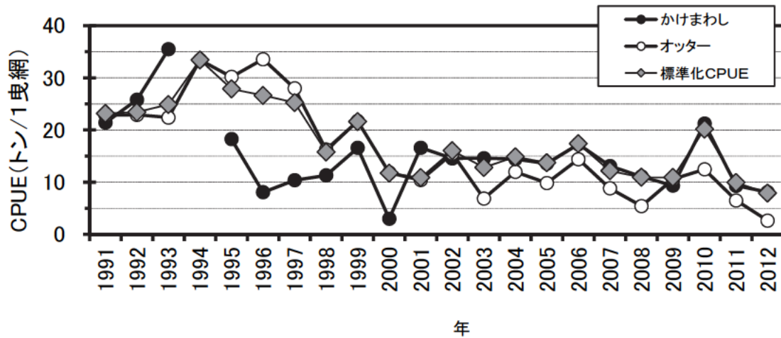
図5 イカナゴ専獲(80%以上)条件により抽出された CPUE および標準化 CPUE の推移
