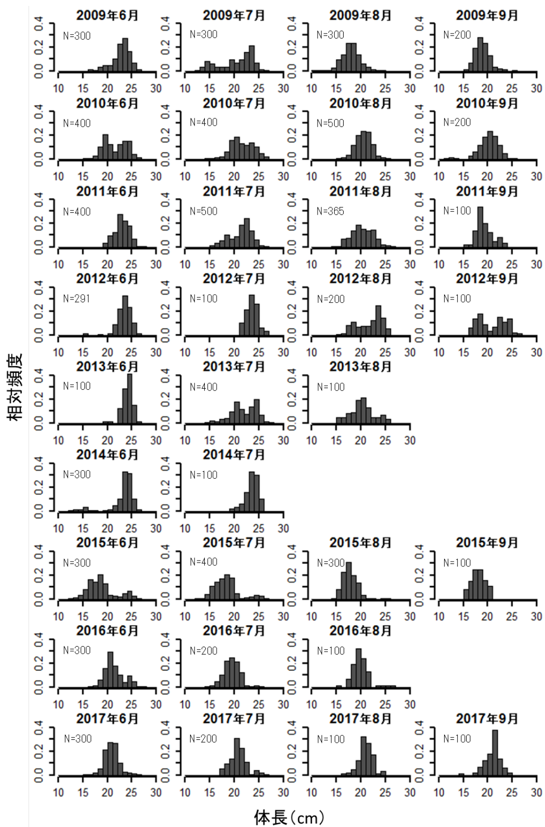
図4 稚内港根拠沖合底びき網漁業によるイカナゴ類漁獲物の月別体長組成 (N: 測定尾数)
