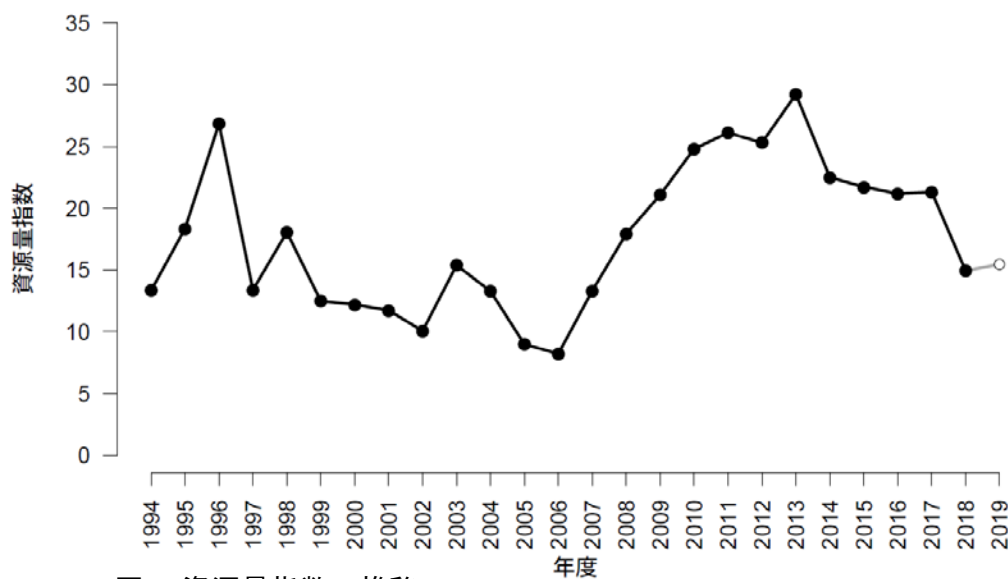
図6 資源量指数の推移.
