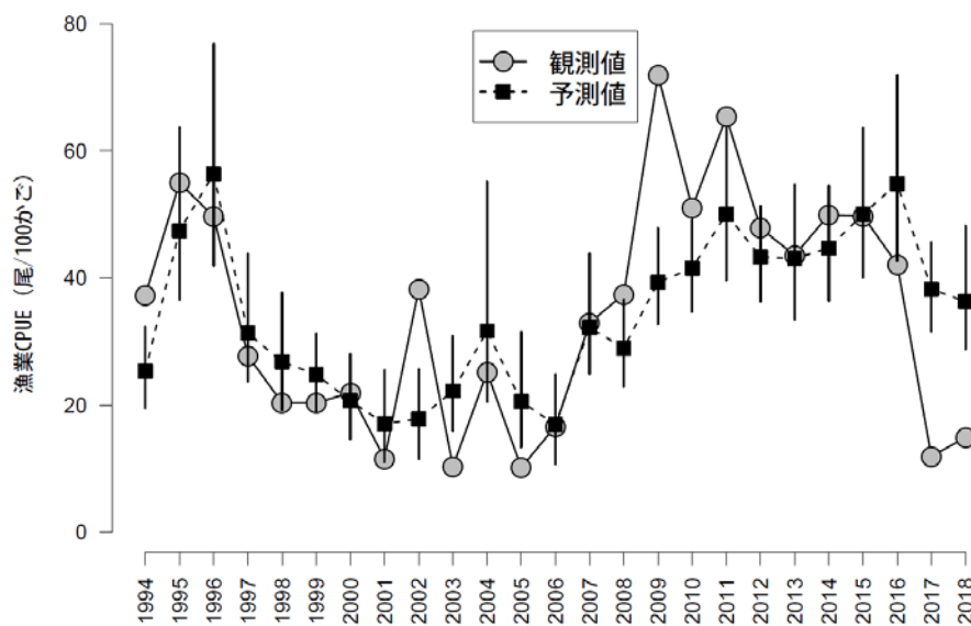
図4 漁業 CPUE 観測値と予測値のあてはめ結果.
