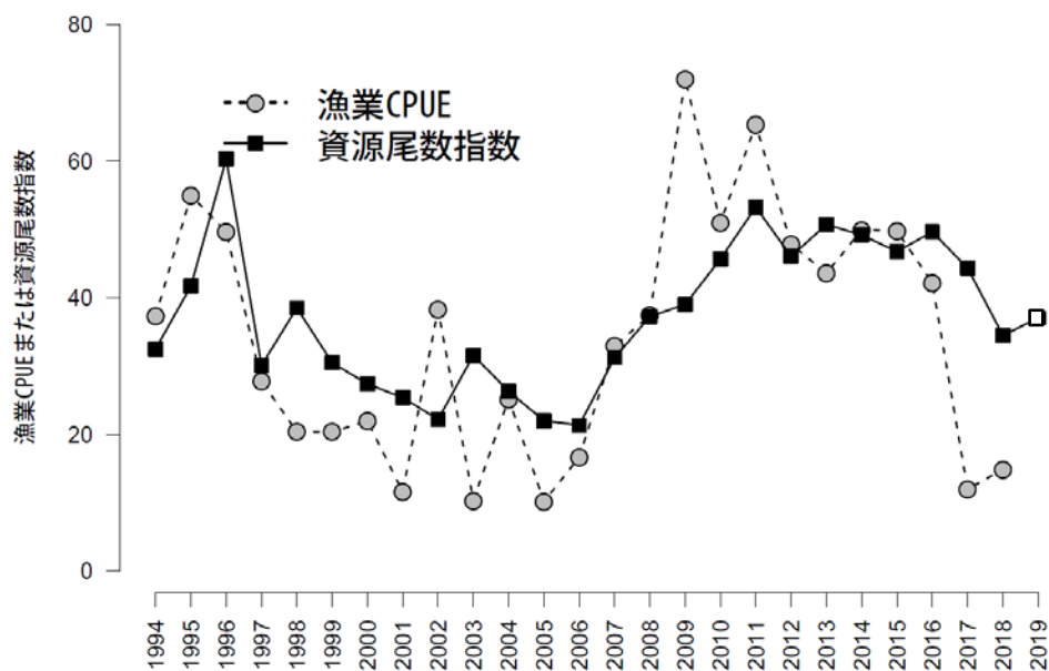
図5 資源尾数指数(標準化 CPUE)と漁業 CPUE の推移.
