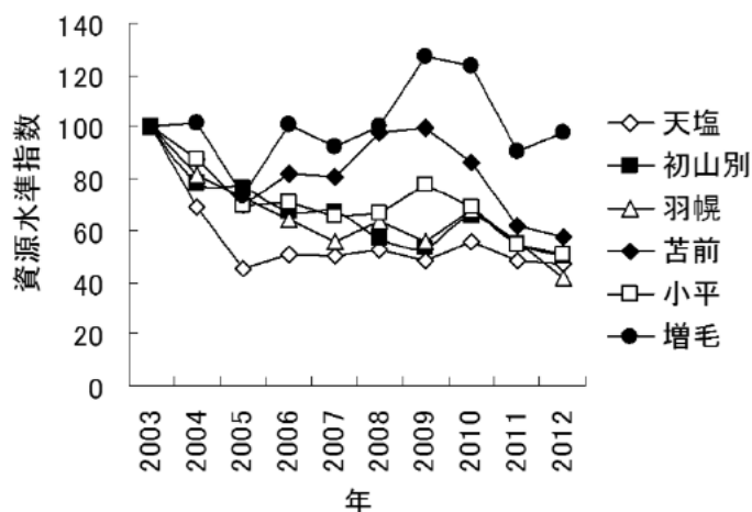
図9 留萌管内における地区別のたこ箱CPUEの経年変化 2003年のたこ箱CPUE (kg/(日・隻)) を100としたときの相対値
