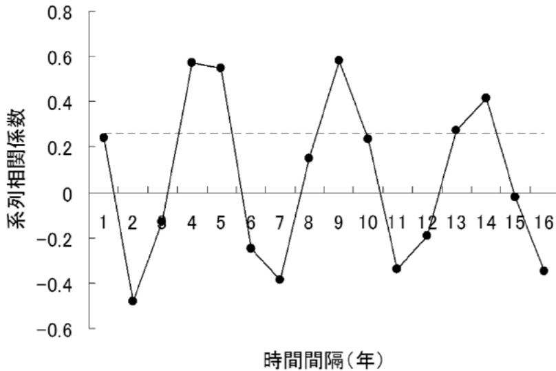
図6 宗谷地区のたこいさり樽流しCPUEのコレログラム データは1982年から2012年の31年分,2年以上の時間間隔で p < 0.05
