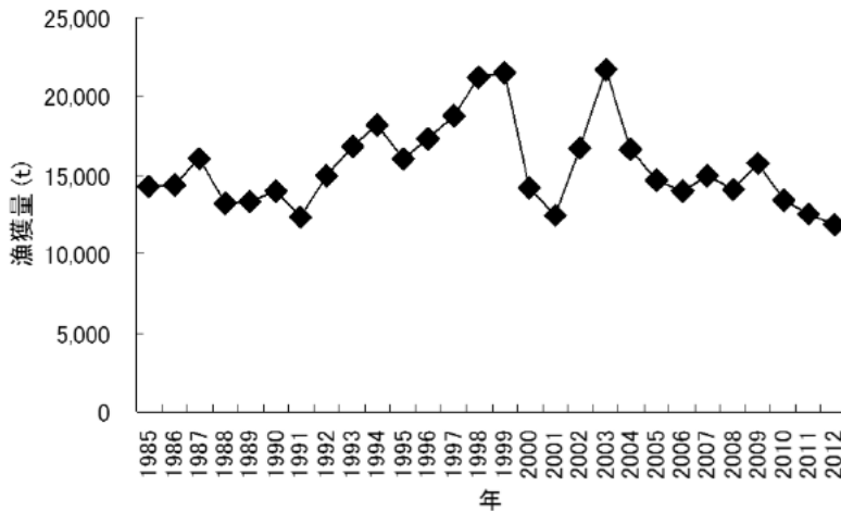
図2 北海道のミズダコ漁獲量の推移 2012年は水試集計速報値
