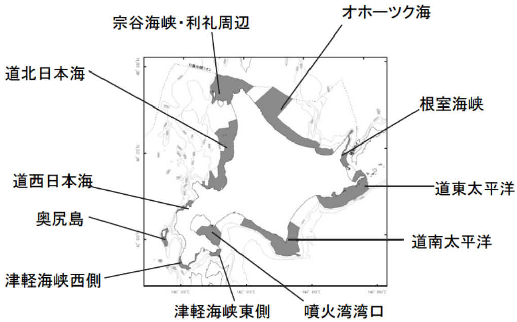
図1 北海道におけるミズダコ資源評価のための海域区分 黒塗り範囲が資源評価海域
