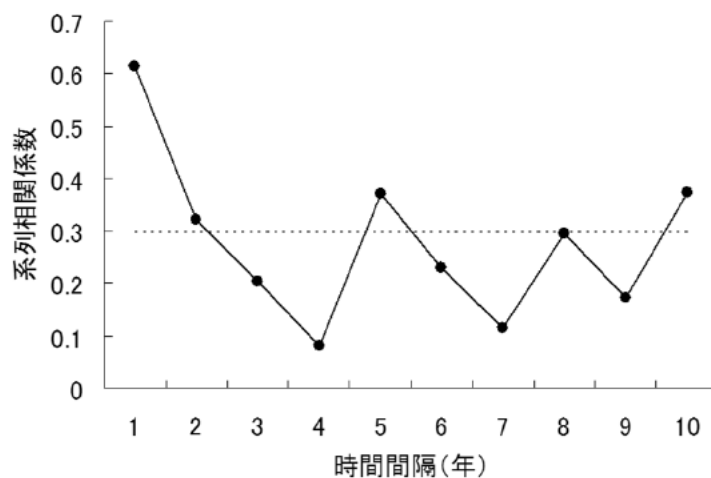
図8 留萌管内増毛地区におけるたこ空つり縄CPUEのコレログラム データは1993年から2012年の20年分、 p < 0.05
