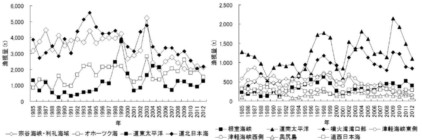
図3 資源評価海域別のミズダコ漁獲量の推移 左図：漁獲量の最高値が2000t以上の海域，右図：漁獲量の最高値が2000t未満の海域 2012年は水試集計速報値
