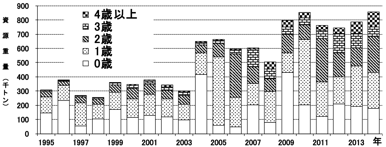
図6 ゴマサバ太平洋系群年齢別資源重量(千トン, 漁期年:7月1日~6月30日)
