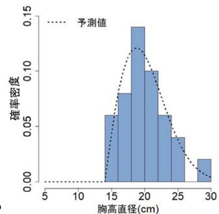
図-2 直径分布のヒストグラムと、ワイブル分布のあてはめの例
