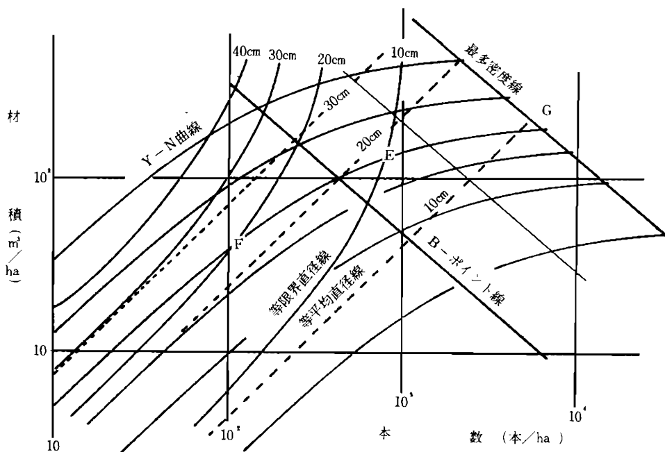
図—5 ミズナラ林の収量—密度図
