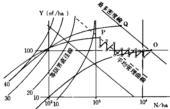
図-8 模型的な間伐径路図
