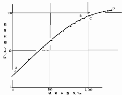
図一 6 積算材積と積算本数の関係 (表一2の資料を両対数グラフにプ ロットしたもの) 曲線はY-N曲線である。
