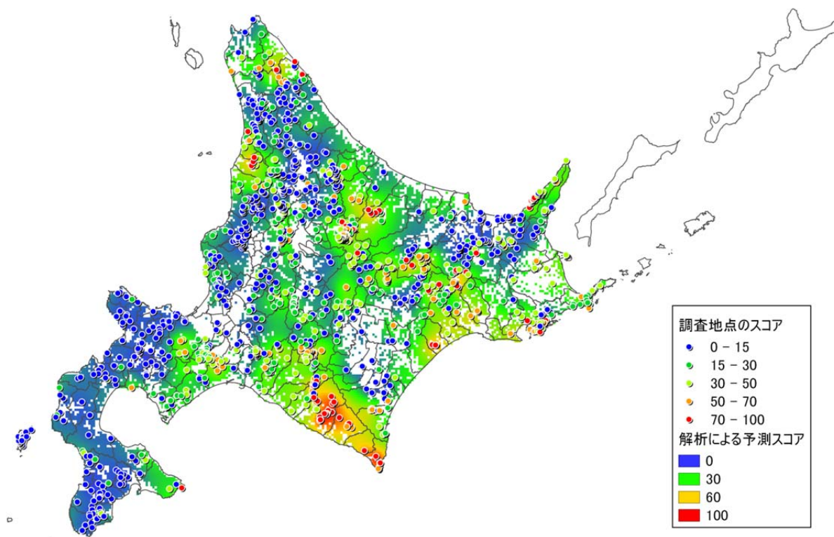
図－２ 簡易チェックシートによる天然林の評価結果
