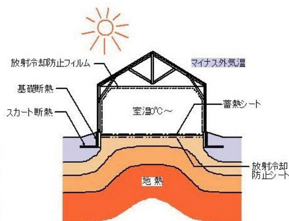
図4 冬期間の木造無加温温室のイメージ
