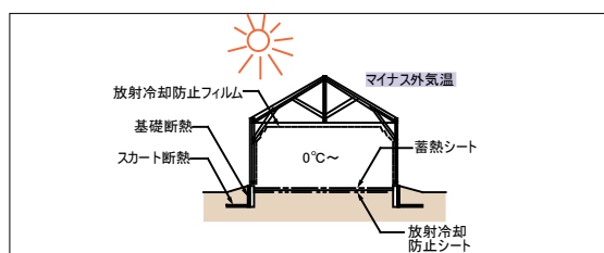
CASE I 仮設型温室からの脱却を図る 基礎断熱工法を採用したセルフビルドによる木造無加温温室
