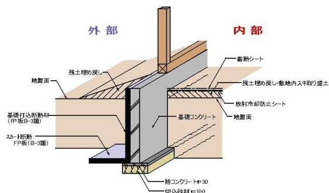
図3 基礎断熱の工法
