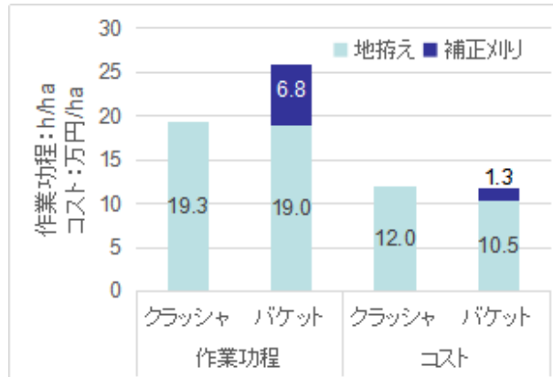
図-3 クラッシュ、バケット地拵えの 作業工期とコストの比較
