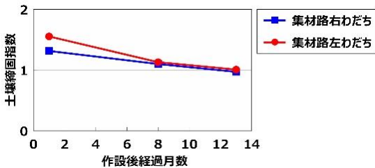
図-2 月形における作業道作設経過月数と土壌締固め指数の関係
