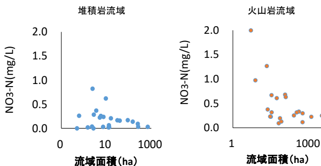
図-1 地質の異なる2流域における流域面積と平水時の硝酸態窒素( \text{NO}_3\text{-N} )濃度の関係
