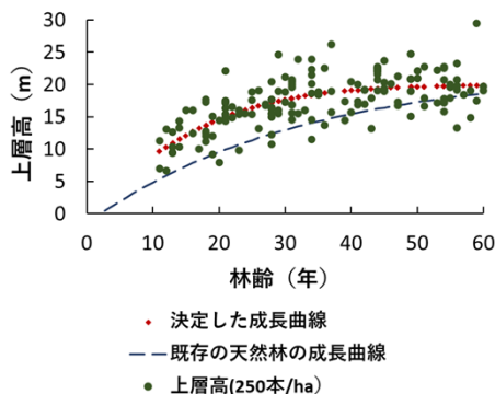
図-1 林齢と上層高の関係における各成長曲線のあてはめおよび50年生時の上層高
