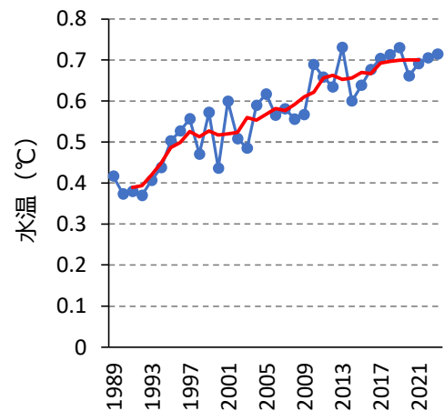
図 2 定期海洋観測で記録された留萌沖水深 500m の水温推移
