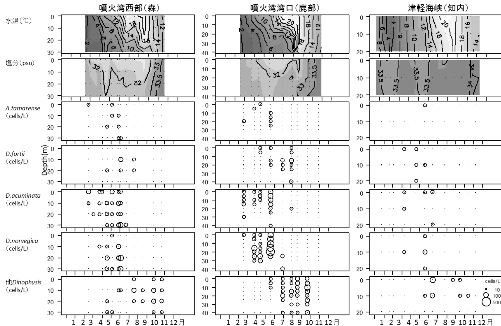
図8 噴火湾西部(森)、同湾口(鹿部)、津軽海峡(知内)海域における水温・塩分と A. tamarense および Dinophysis 属の鉛直分布の季節変化
